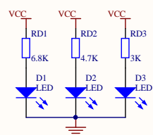
电源指示灯
