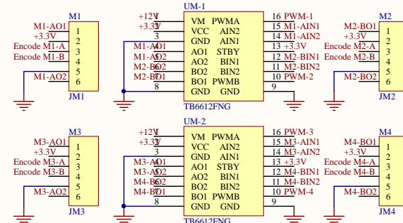
电机驱动
