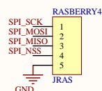
树莓派通讯
