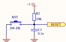
复位电路
