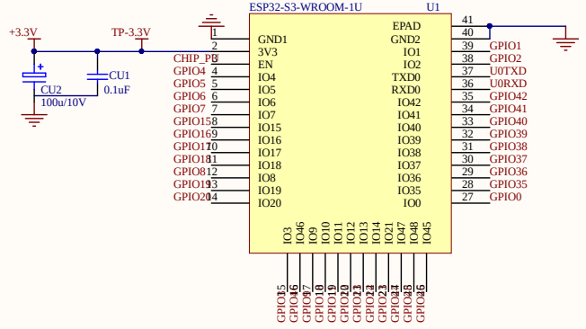
MCU ESP32-S3
