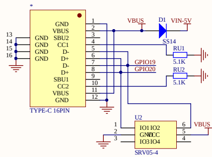
USB JTAG
