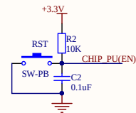
RST
