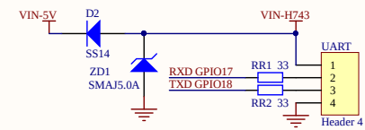
UART
