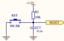
复位电路
