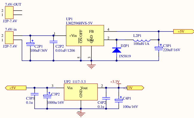
电源电路
