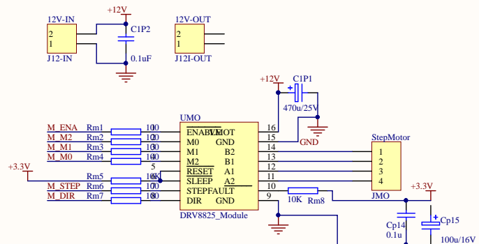
DRV8825
