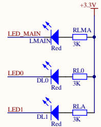
LED指示灯
