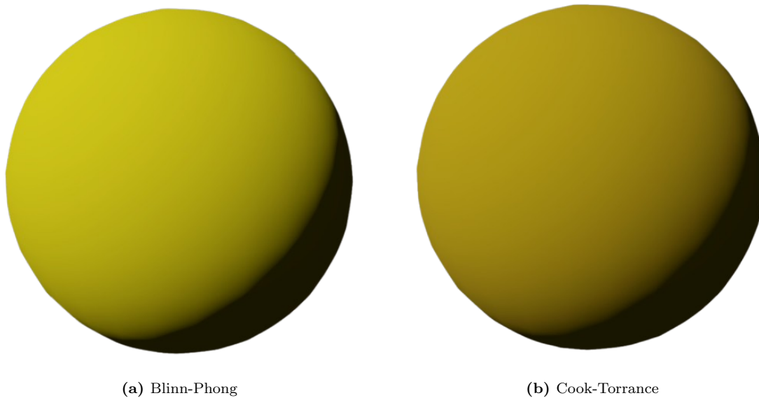
Figura 5.8: Confronto con rugosità elevata. In Cook-Torrance i bordi risultano più scuri per effetto del termine G , assente in Blinn-Phong.
