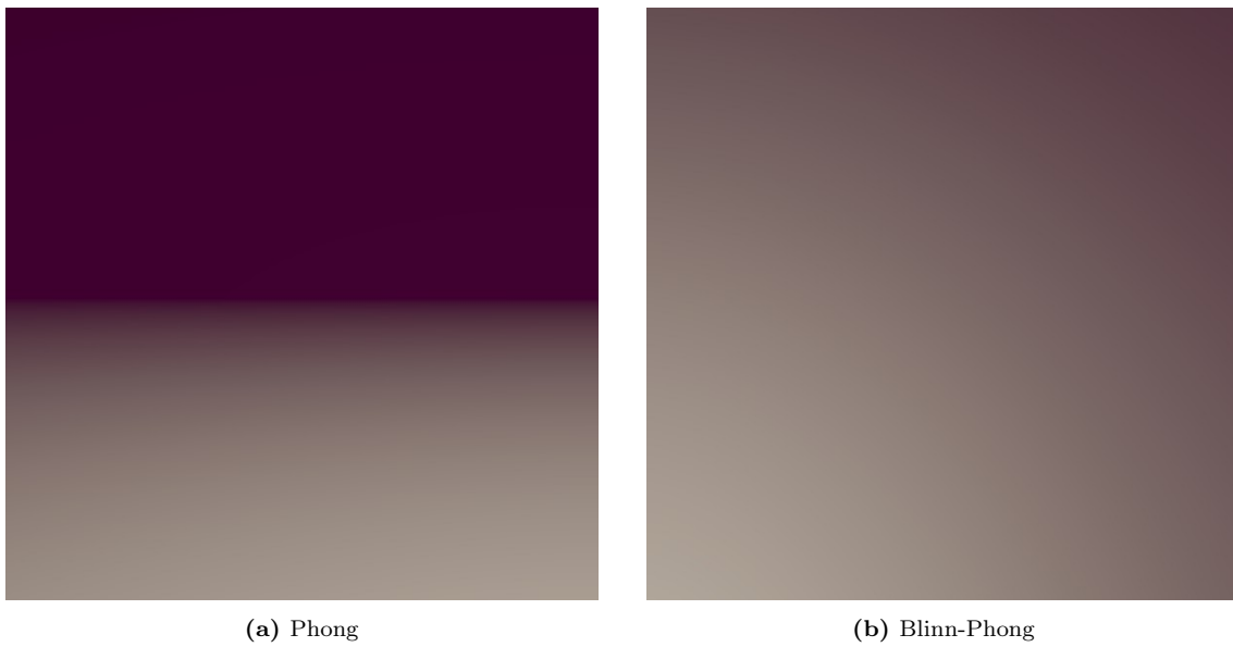
Figura 5.6: Lo stesso confronto su un piano, visto dall'alto con la sorgente luminosa alle spalle dell'osservatore. Il taglio netto del riflesso di Phong è ancora più evidente che sulla sfera.
