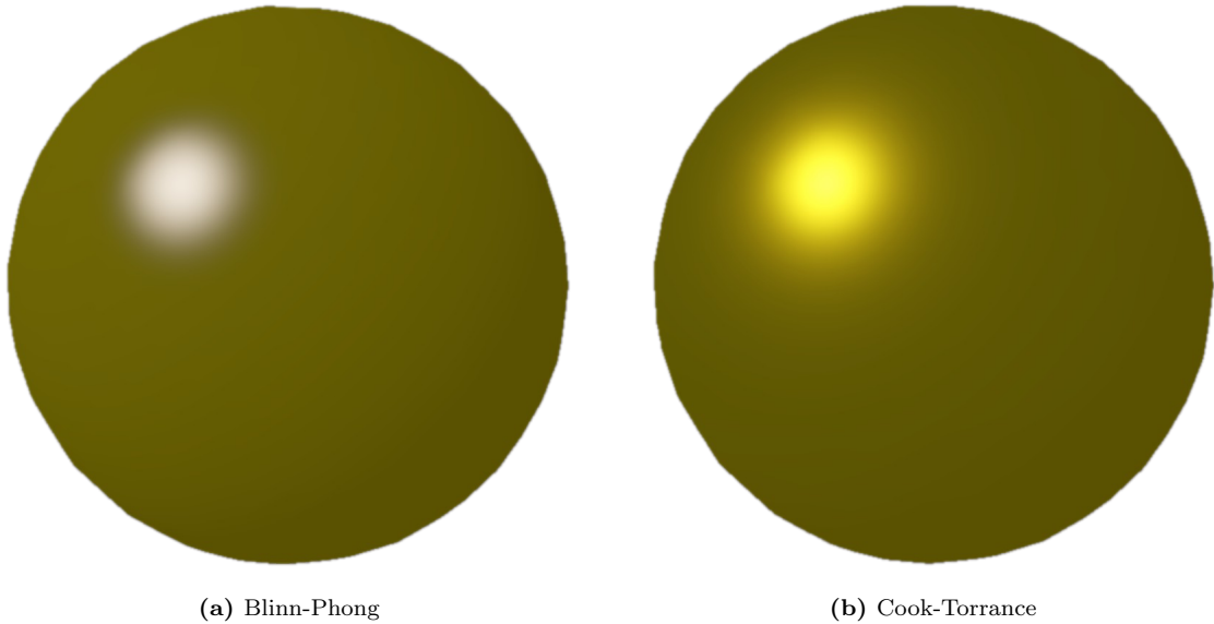
Figura 5.7: Confronto su un materiale metallico (oro). In Blinn-Phong il riflesso speculare è bianco; in Cook-Torrance assume il colore dell'albedo.
