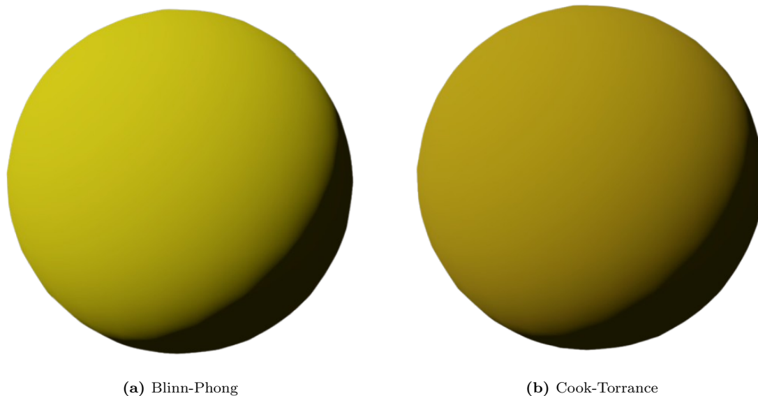
Figura 5.7: Confronto con rugosità elevata. In Cook-Torrance i bordi risultano più scuri per effetto del termine G , assente in Blinn-Phong.
