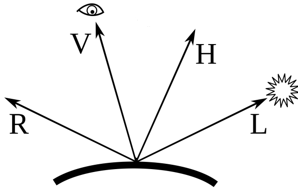
Figura 2.4: Vettori coinvolti nel modello di Blinn-Phong. Immagine adattata da [Wik] .
