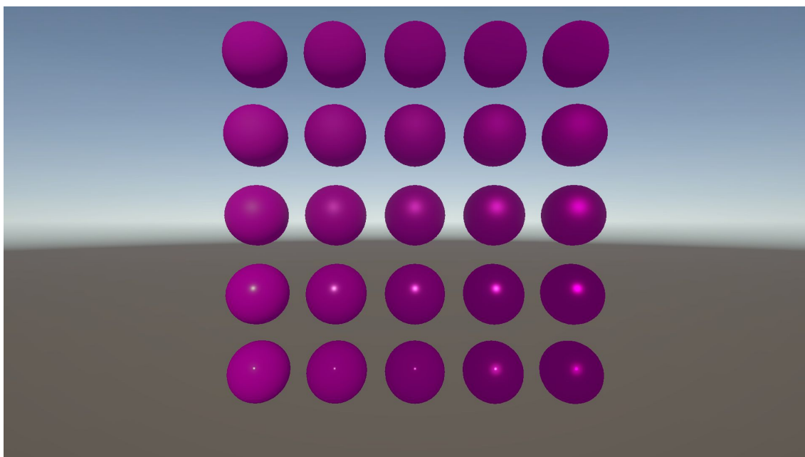
Figura 5.8: Griglia di sfere Cook-Torrance: il metallic cresce da sinistra a destra, la roughness dal basso verso l'alto.
