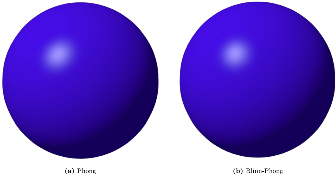
Figura 5.4: Confronto tra Phong e Blinn-Phong con parametri equiparati. In condizioni ordinarie i due modelli sono quasi indistinguibili.
