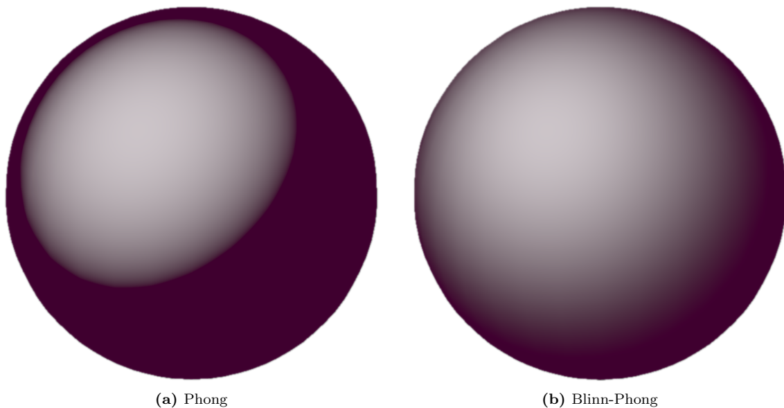
Figura 5.5: Riflesso speculare su una sfera con shininess molto bassa. In Phong il riflesso presenta un taglio netto, assente in Blinn-Phong.
