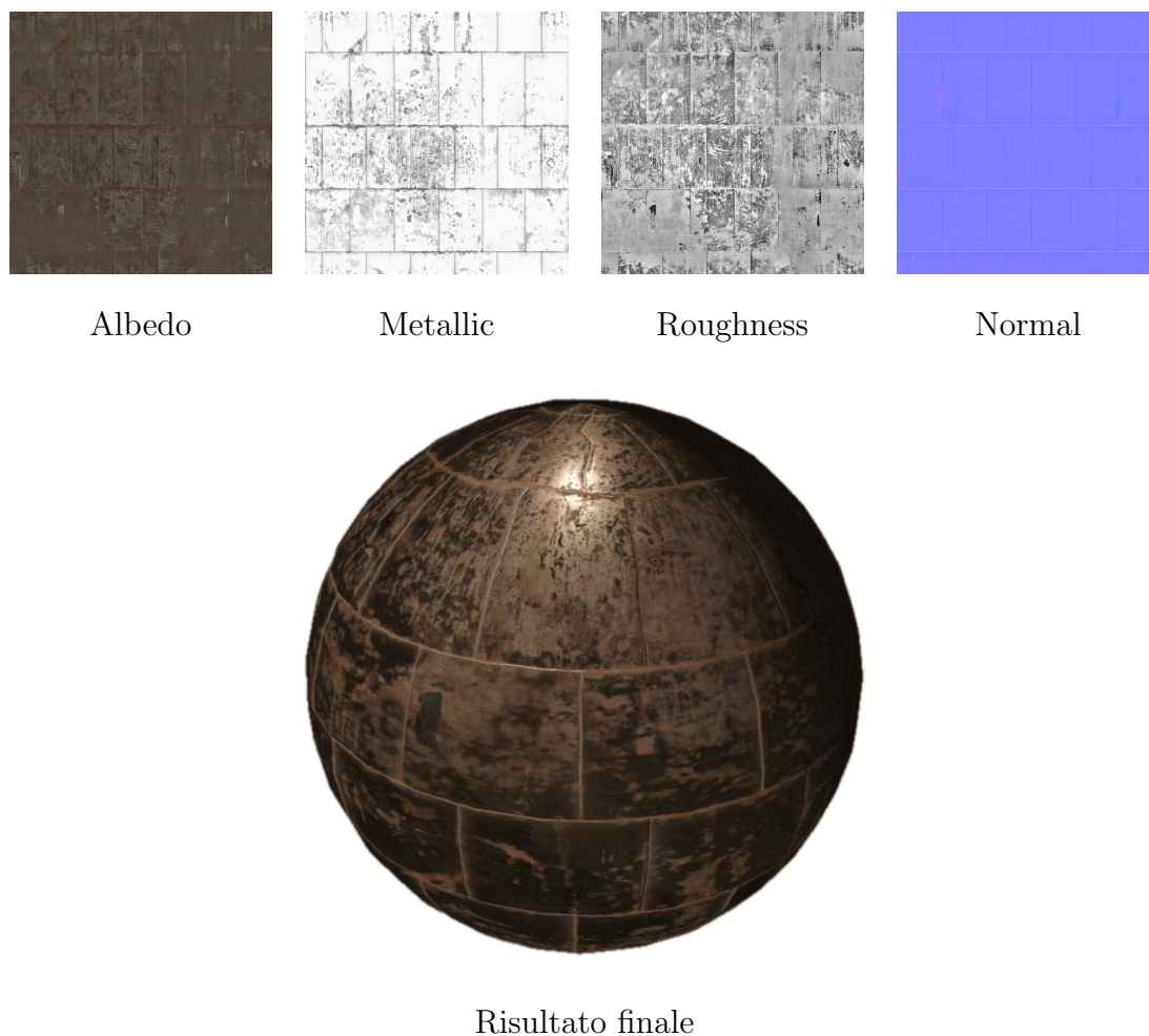
Figura 3.8: Le texture map e il risultato della loro combinazione nel modello di Cook-Torrance.
