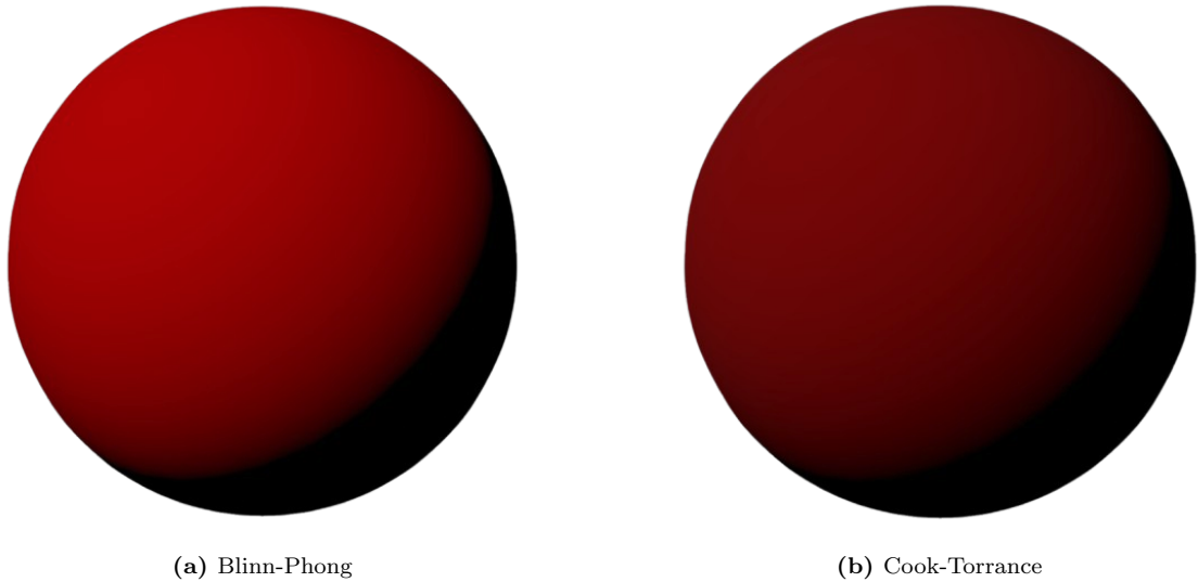
Figura 5.9: Confronto con rugosità elevata. In Cook-Torrance i bordi risultano più scuri per effetto del termine G , assente in Blinn-Phong.
