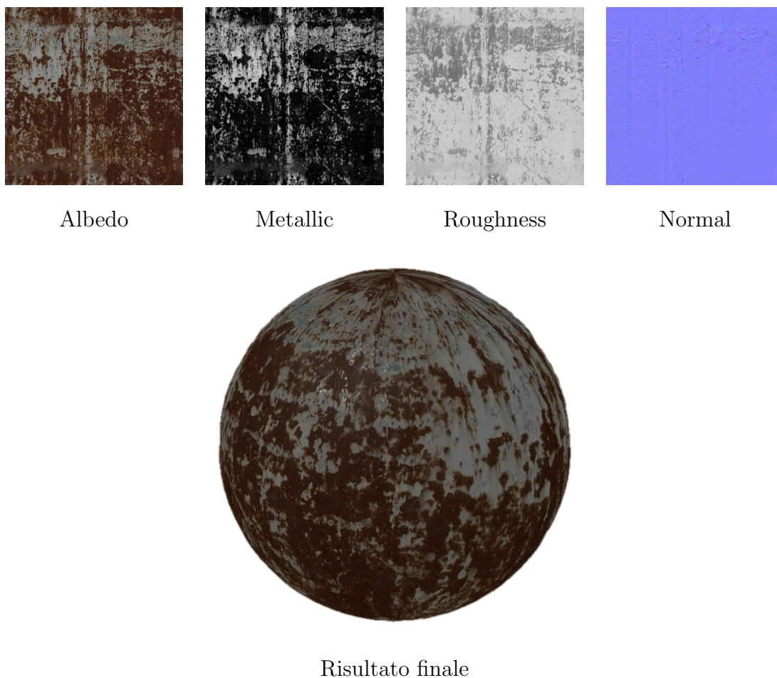
Figura 3.8: Le texture map e il risultato della loro combinazione nel modello di Cook-Torrance.
