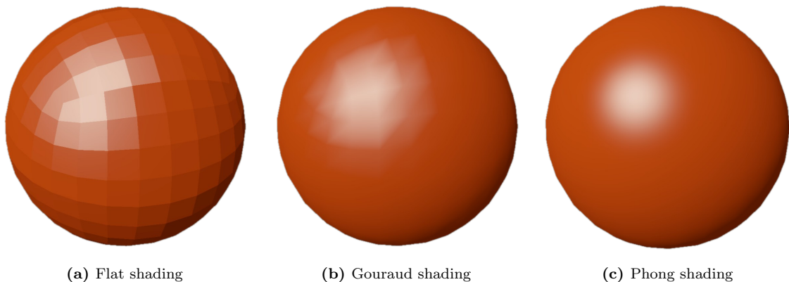
Figura 2.7: Confronto tra le tre tecniche di shading applicate a una sfera a bassa risoluzione.
