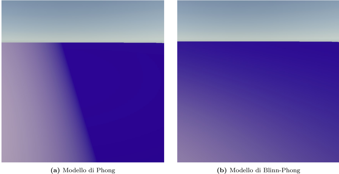
Figura 2.6: Riflesso speculare su un piano con luce radente e un valore di shininess basso. Nel modello di Phong il riflesso presenta un taglio netto, assente in Blinn-Phong.
