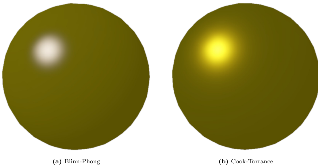
Figura 5.8: Confronto su un materiale metallico (oro). In Blinn-Phong il riflesso speculare è bianco; in Cook-Torrance assume il colore dell'albedo.
