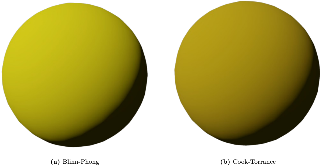
Figura 5.9: Confronto con rugosità elevata. In Cook-Torrance i bordi risultano più scuri per effetto del termine G , assente in Blinn-Phong.
