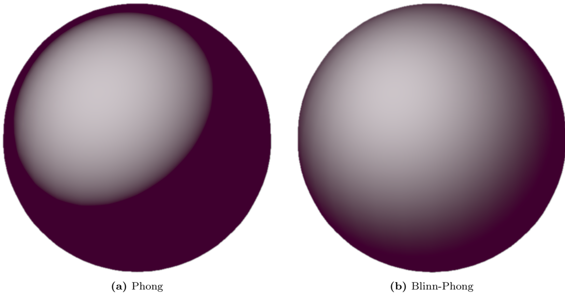
Figura 5.6: Riflesso speculare su una sfera con shininess molto bassa. In Phong il riflesso presenta un taglio netto, assente in Blinn-Phong.
