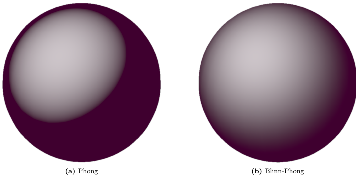
Figura 5.6: Riflesso speculare su una sfera con shininess molto bassa. In Phong il riflesso presenta un taglio netto, assente in Blinn-Phong.
