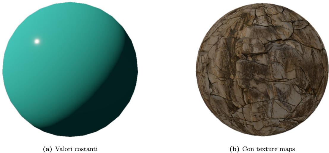
Figura 5.12: Lo stesso modello Cook-Torrance con valori costanti e con texture maps. Le texture permettono di variare i parametri del materiale punto per punto.
