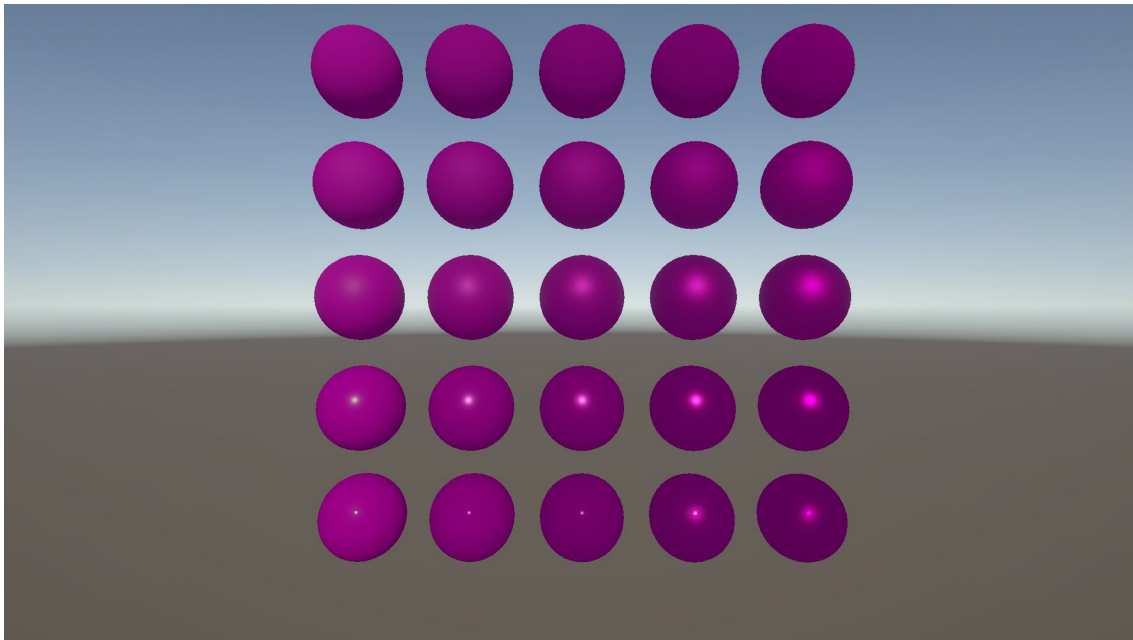
Figura 5.11: Griglia di sfere Cook-Torrance: il metallic cresce da sinistra a destra, la roughness dal basso verso l'alto.
