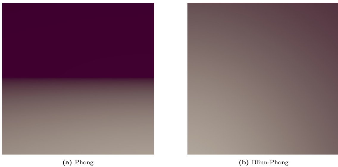
Figura 5.7: Lo stesso confronto su un piano, visto dall'alto con la sorgente luminosa alle spalle dell'osservatore. Il taglio netto del riflesso di Phong è ancora più evidente che sulla sfera.
