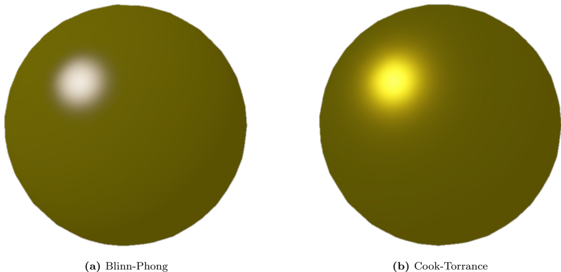
Figura 5.8: Confronto su un materiale metallico (oro). In Blinn-Phong il riflesso speculare è bianco; in Cook-Torrance assume il colore dell'albedo.
