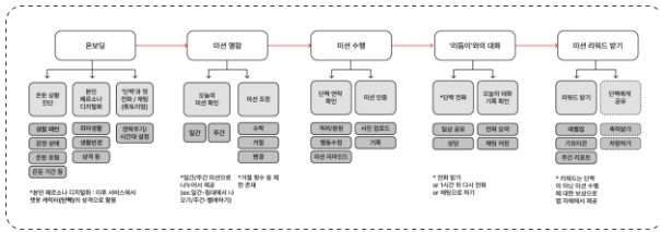
그림 1 Task Flow
