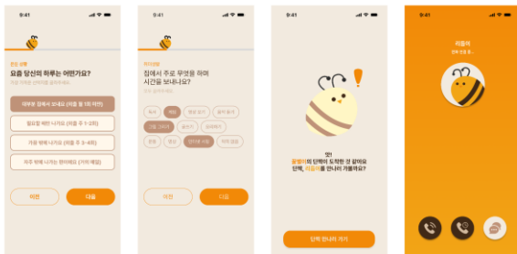
그림 2 온보딩 프로세스
