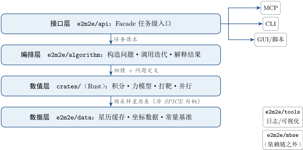
图 1: e2m2e 运行时分层。依赖单向向下: 接口层同源派生 CLI/MCP; 编排层只构造问题不做迭代; Rust 数值层不持有 SPICE 句柄, 星历以预采样缓存表注入。
