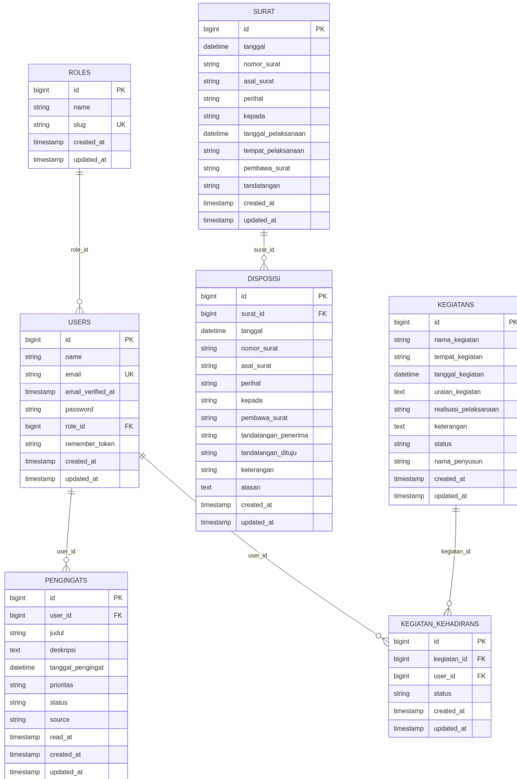
Gambar: Rancangan Database (ERD)
