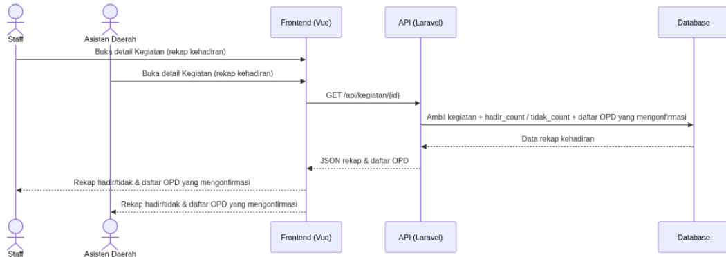
Gambar: Sequence Diagram Lihat Rekap & Daftar OPD
