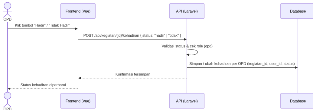
Gambar: Sequence Diagram Konfirmasi Kehadiran
