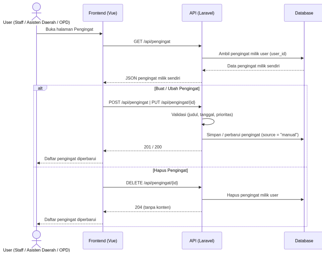
Gambar: Sequence Diagram Kelola Peningat Pribadi
