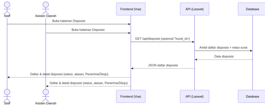
Gambar: Sequence Diagram Lihat Disposisi
