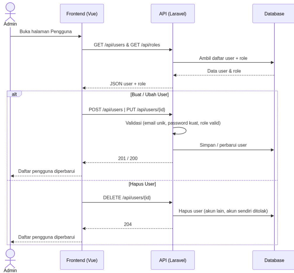
Gambar: Sequence Diagram Kelola Pengguna & Role
