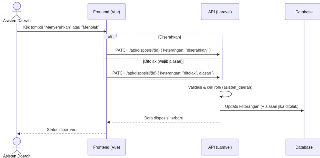
Gambar: Sequence Diagram Asisten Daerah Meninjau Disposisi
