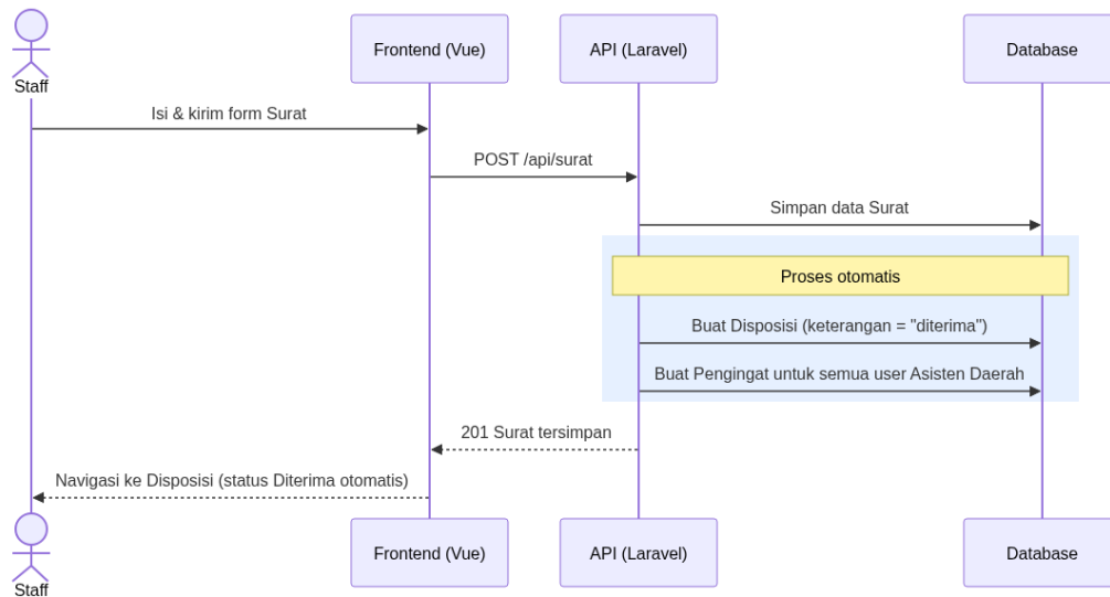
Gambar: Sequence Diagram Staff Membuat Surat
