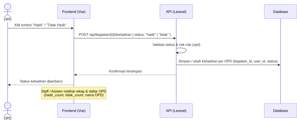
Gambar: Sequence Diagram Konfirmasi Kehadiran
