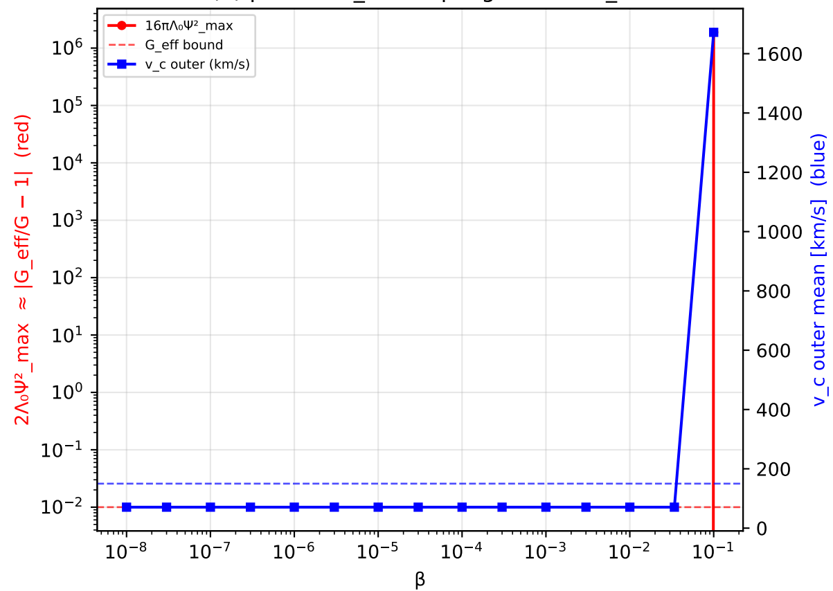
(d) \beta scan: G_{\text{eff}} coupling & outer v_c
