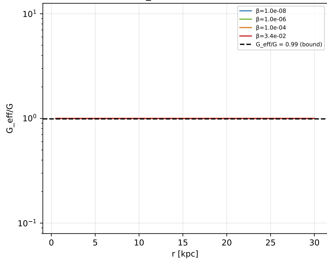
(d) \beta scan: G_{\text{eff}} coupling & outer v_c
