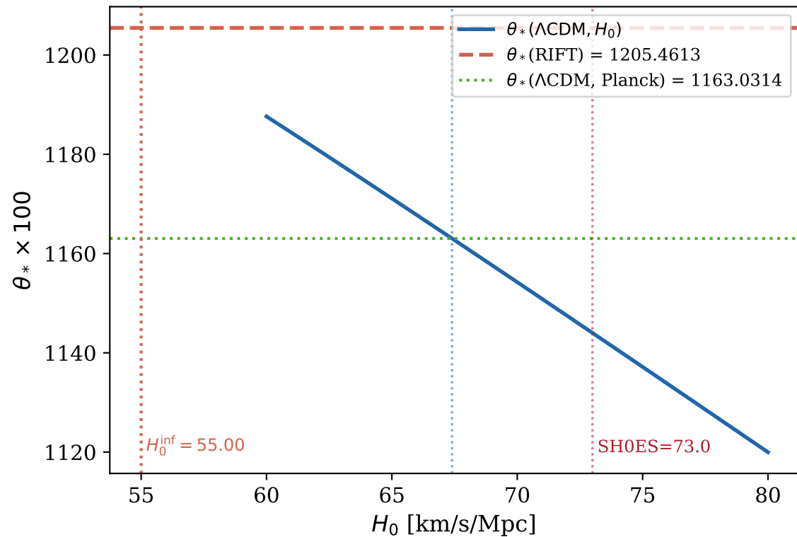
CMB Acoustic Scale: RIFT vs \Lambda CDM
