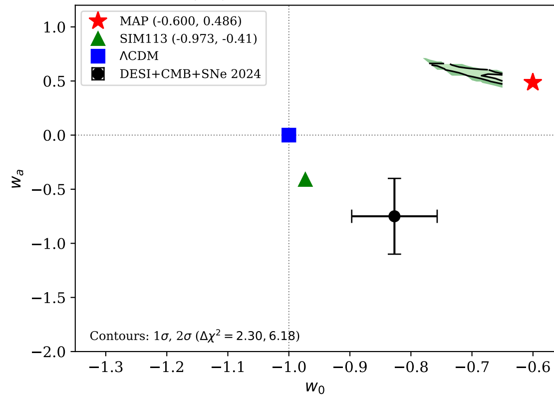
w_0 - w_a Posterior (RIFT MAP F_0 )
