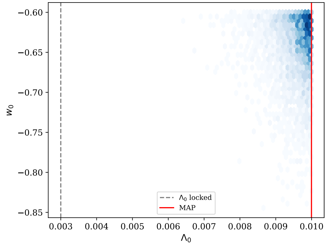
Posterior: \Lambda_0 vs w_0
