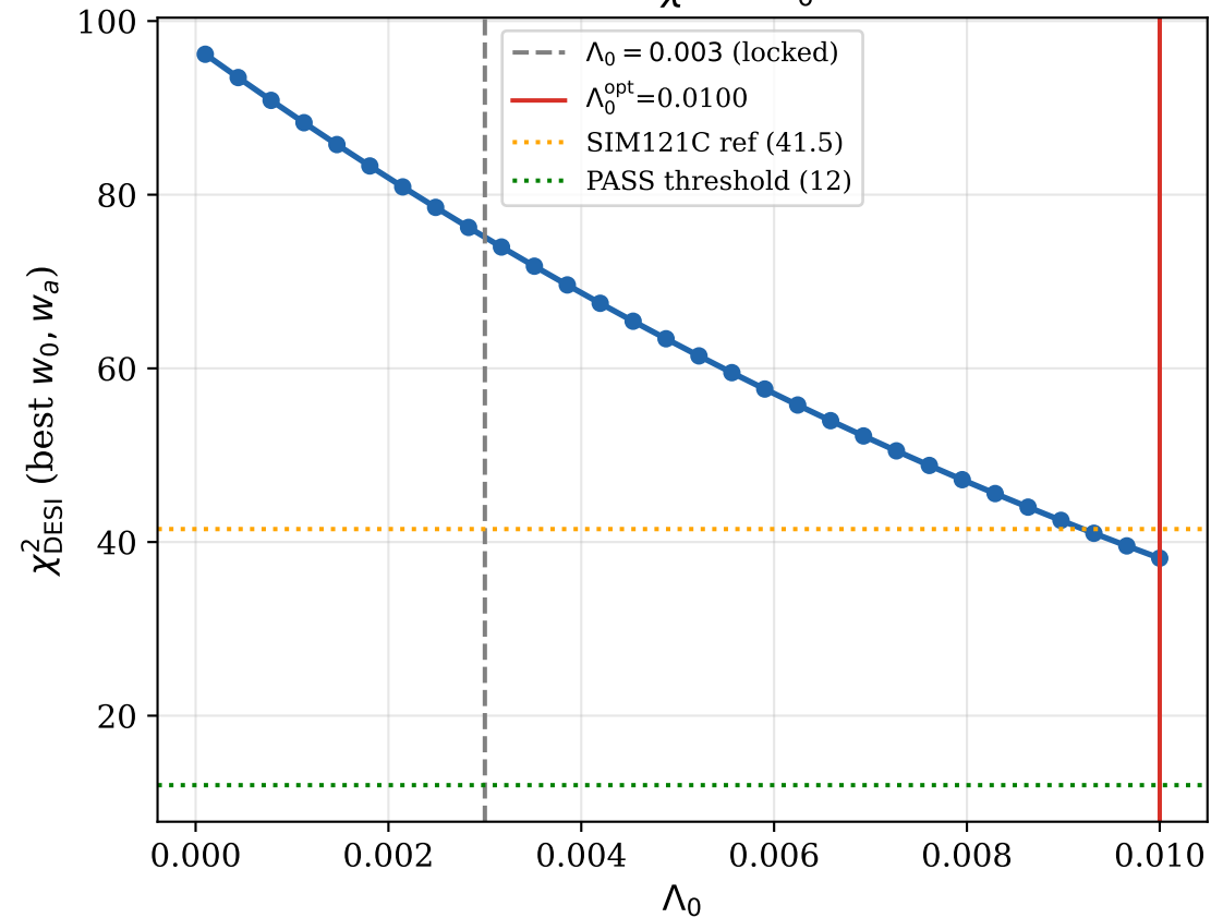
DESI \chi^2 vs \Lambda_0
