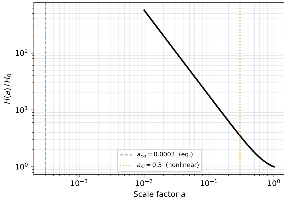
Panel 1 — Hubble Parameter
