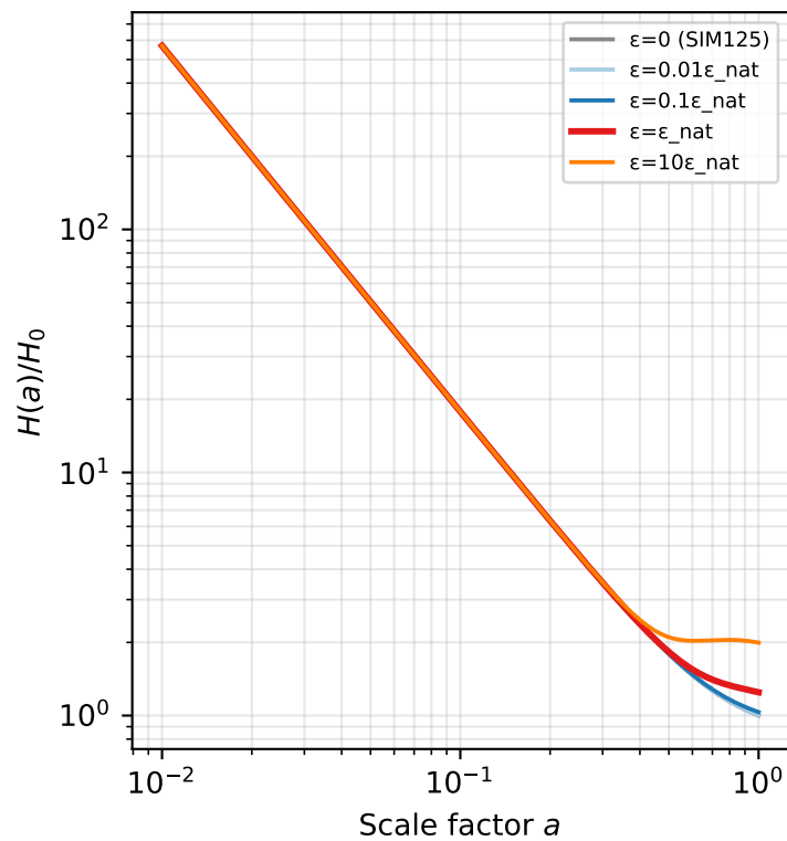
Panel 1 — Hubble Parameter
