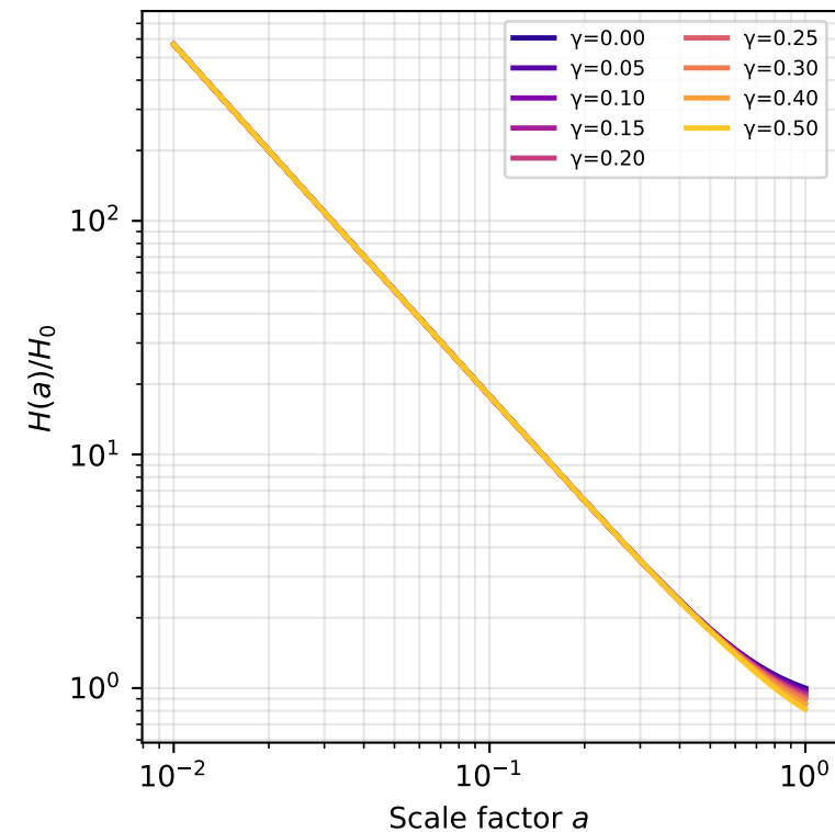
Panel 3 — Hubble Parameter
