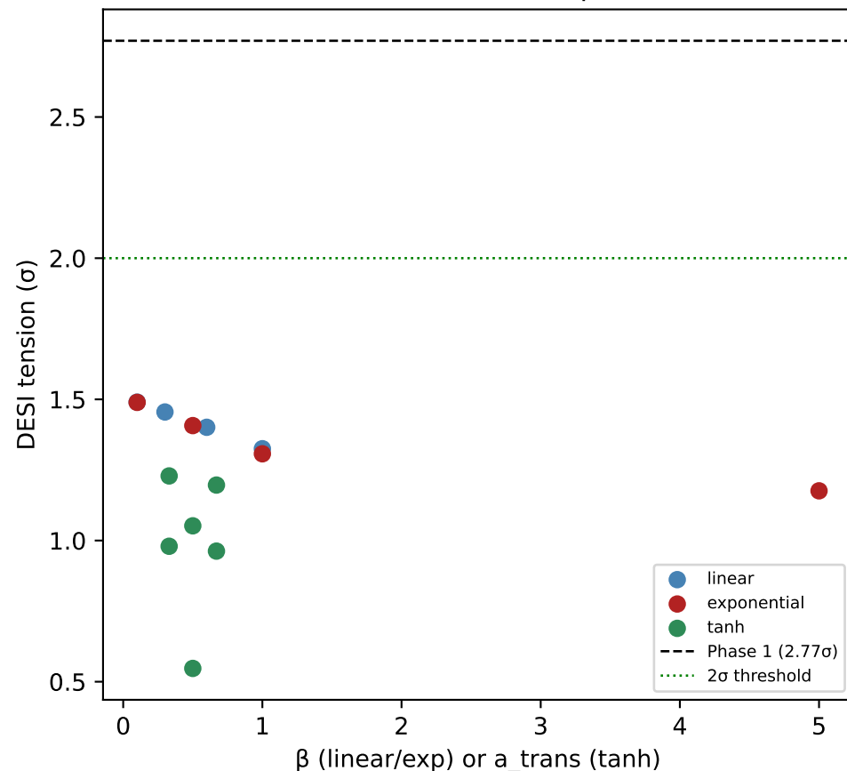
SIM141: DESI tension vs parameter
