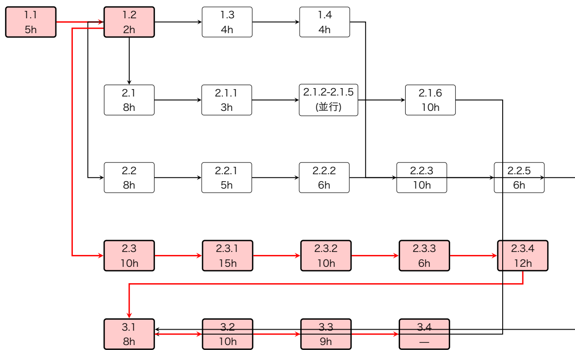
図 1.1: WBS アローダイアグラム (赤色がクリティカルパス)
