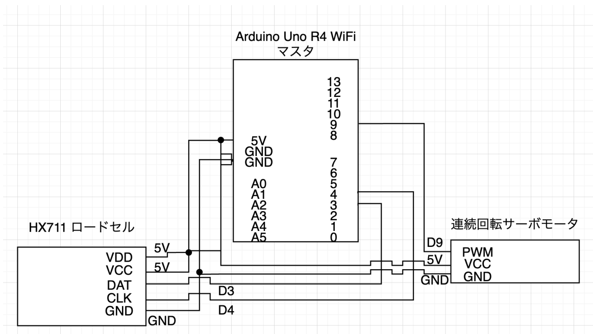
図 3.3: マスタとロードセル・連続回転サーボモーターを接続した回路図
