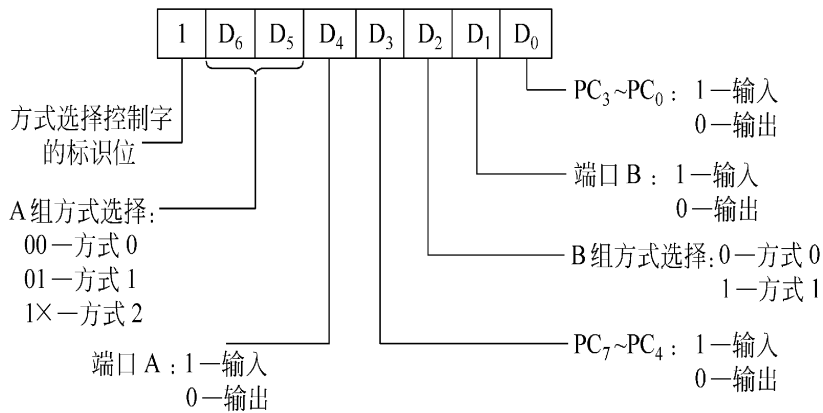
8255 初始化命令字
