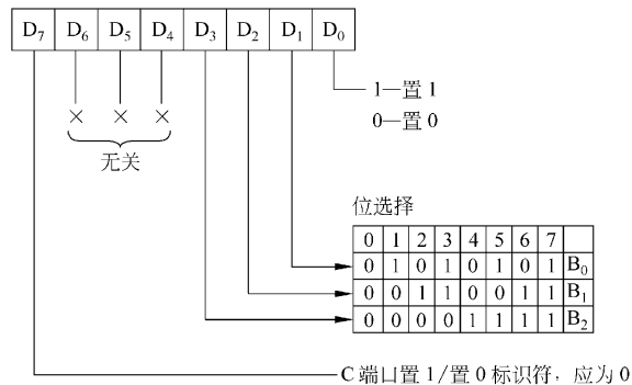
8255 C 口置位复位控制字
