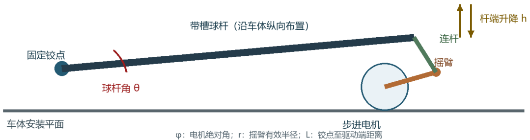
图 2 步进电机摇杆带动球杆单端升降的结构示意
