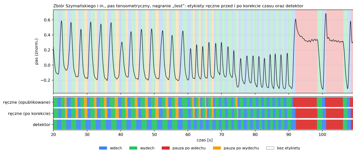
Rysunek 13.10: Nagranie pasa ze zbioru [26]. Tło: etykiety ręczne po korekcie czasu; paski: etykiety opublikowane, po korekcie i detektor deterministyczny. Po korekcie granice leżą na zwrotach pasa, a pauza po wdechu zaczyna się w szczycie; szybkie osiadanie tuż po nim należy do pauzy, zarówno w etykietach, jak i w detektorze. Krótkie pauzy po wydechu detektor wlicza do wydechu.
