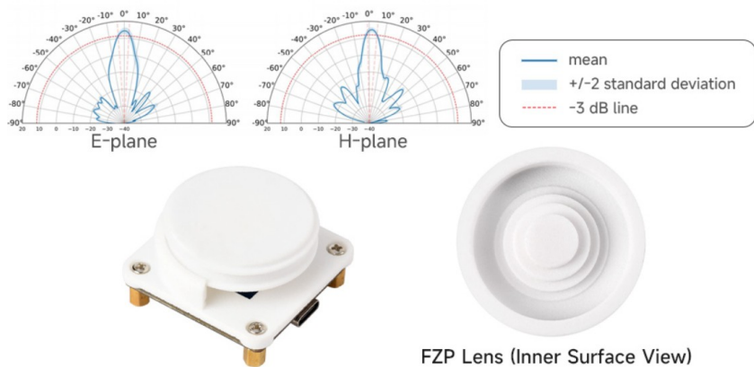
(b) Soczewka FZP — porównywalny zysk, wyraźniej silniejsze listki boczne.
