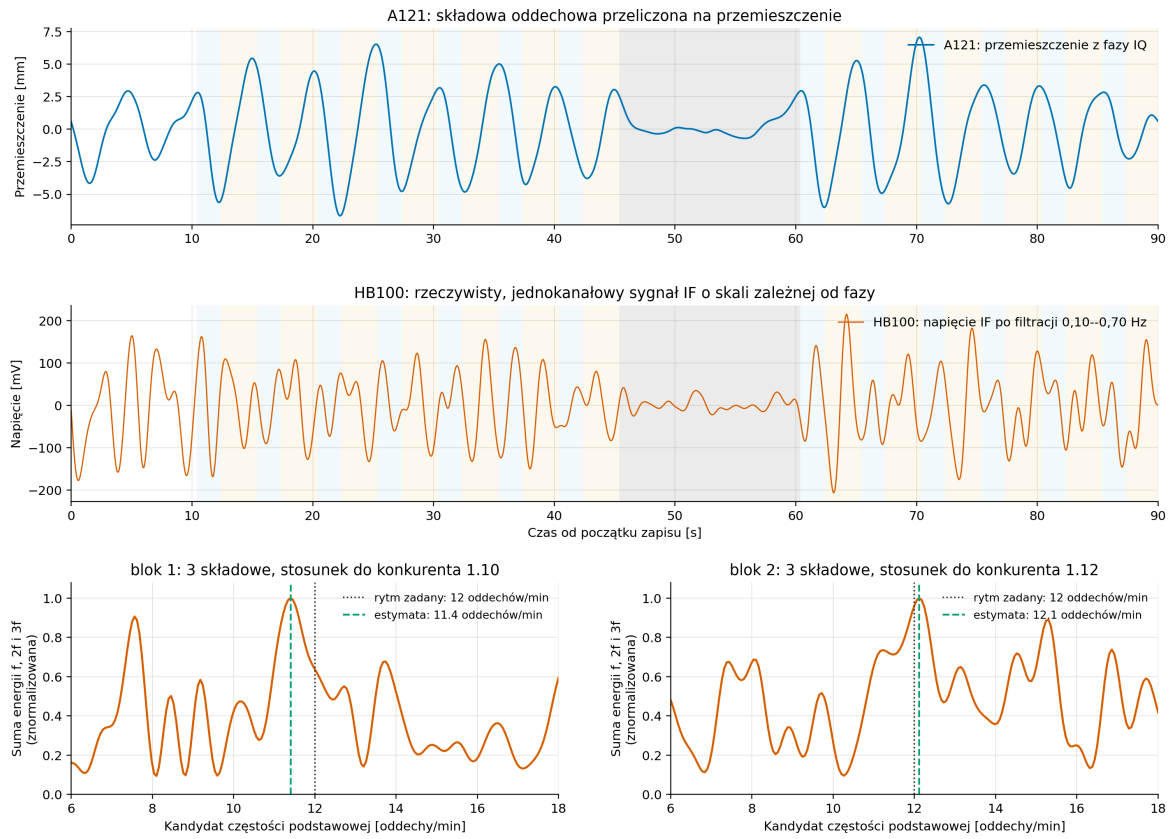
Rysunek 11.4: Pojedynczy retest na 150 cm, wyodrębniony z powtarzanej serii ze względu na brak powtórzenia. Górny panel pokazuje przemieszczenie wyznaczone z fazy IQ A121, środkowy — jednokanałowe napięcie IF HB100; zachowano osobne jednostki, aby nie sugerować ich równoważności. Dolne panele pokazują funkcję (11.2): mimo najsilniejszych pików napięcia przy około 0,37 Hz, estymator wskazał 0,190 Hz (11,4 oddechów/min) oraz 0,202 Hz (12,1 oddechów/min) wobec zadanego rytmu 0,20 Hz. Marże jakości 2,9 i 2,1 są jednak blisko progu akceptacji 2,0; pojedynczy retest stanowi więc jedynie graniczne wskazanie rytmu, a nie podstawę do estymacji fazy wdech–wydech.
