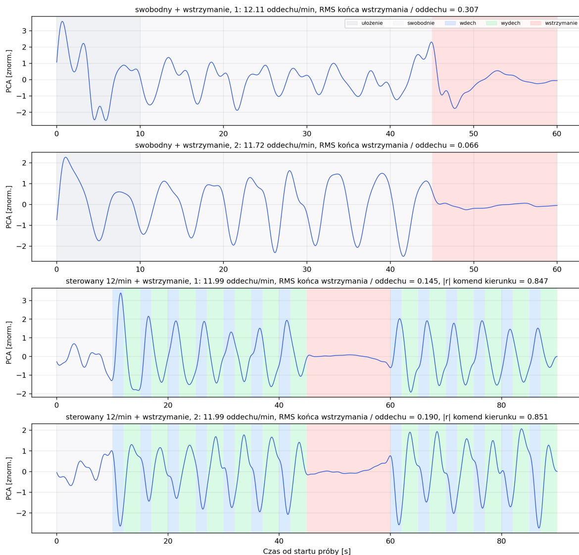
Rysunek 9.3: Znormalizowana pierwsza składowa główna trzech osi przyspieszenia LSM6DS3 po filtracji pasmowej 0,07 Hz do 0,60 Hz. Zacienienie oznacza harmonogram komend; znak PCA jest umowny. Dwa dolne przebiegi odtwarzają rytm 12 oddechów/min, a we wszystkich czterech próbach końcowa część fazy wstrzymania ma wyraźnie mniejszą amplitudę.
