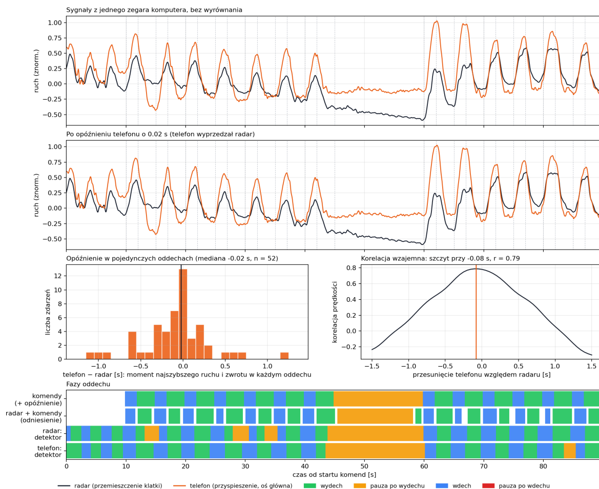
Rysunek 13.4: Lekki oddech z komendami, telefon przy dolnych żebrach. Wykresy górne: sygnały przed wyrównaniem i po nim (linie przerywane to początki komend). Środek: opóźnienie w pojedynczych oddechach i korelacja wzajemna. Dół: fazy z komend, z radaru i komend (odniesienie) oraz z detektora na radarze i na telefonie przesuniętym o opóźnienie. W pauzie po wydechu telefon pozostaje płaski, a radar dryfuje.
