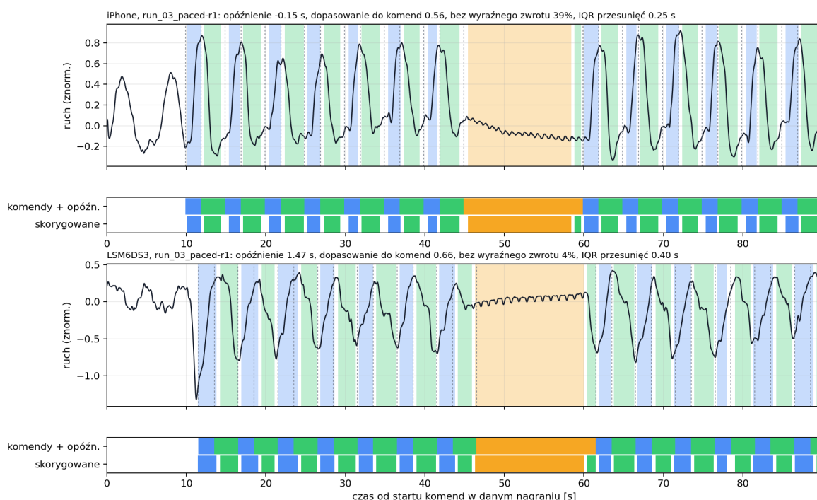
Rysunek 13.3: Etykiety faz wyznaczone tą samą metodą na osobnych nagraniach iPhone’a (góra) i LSM6DS3 (dół), każde względem własnych komend przewodnika.
