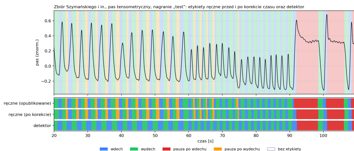
Rysunek 13.7: Nagranie pasa ze zbioru [26]. Tło: etykiety ręczne po korekcie czasu; paski: etykiety opublikowane, po korekcie i detektor deterministyczny. Po korekcie granice leżą na zwrotach pasa, a pauza po wdechu zaczyna się w szczycie; szybkie osiadanie tuż po nim należy do pauzy, zarówno w etykietach, jak i w detektorze. Krótkie pauzy po wydechu detektor wlicza do wydechu.
