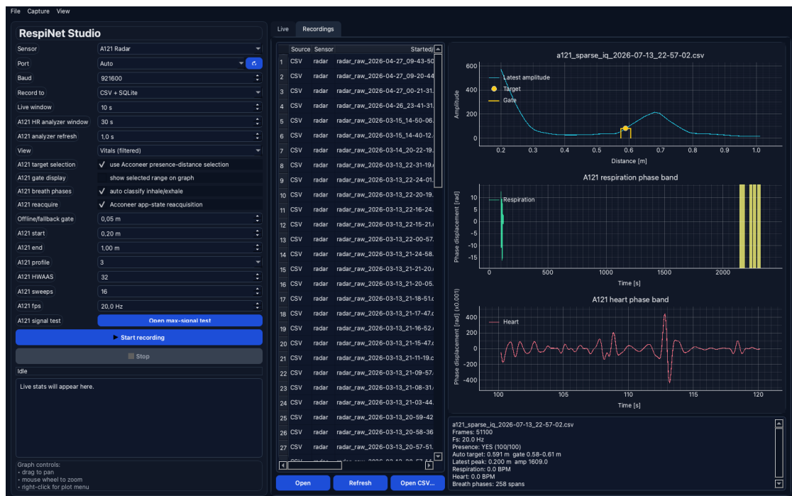
Rysunek 10.5: Przeglądarka nagrań aplikacji desktopowej po otwarciu rzeczywistego pliku Sparse IQ A121. Tabela po lewej pozwala wybrać źródło, a wykresy po prawej pokazują profil amplitudy z bramką oraz składowe oddechową i sercową.
