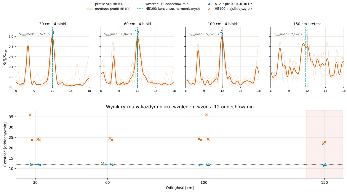
Rysunek 11.3: Porównanie estymacji rytmu we wszystkich 14 blokach. Górny rząd przedstawia funkcję konsensusu harmonicznego S(f) dla HB100: jasne linie są profilami pojedynczych bloków, ciemna — ich medianą dla danego dystansu. Linia kropkowana wyznacza zadane 12 oddechów/min, zielona — medianę estymat HB100, a niebieskie trójkąty — pik 0,10 Hz do 0,30 Hz z A121. Dolny panel pokazuje wynik każdego bloku; krzyżyki to mylące najsilniejsze piki HB100 przed złożeniem harmonicznym. Przy 30 cm do 100 cm profile HB100 mają wyraźniejszą przewagę kandydata przy 12 oddechach/min ( S_{\max}/\text{med } S = 5,7\text{--}21,5 ) niż w pojedynczym reteście 150 cm (2,1–2,9).
