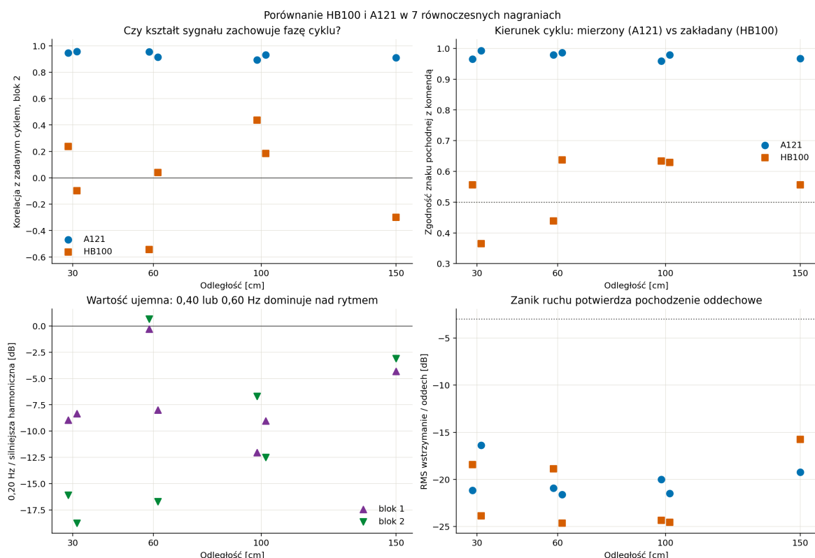
Rysunek 11.5: Metryki sześciu prób podstawowych oraz pojedynczego retestu 150 cm. Dwa górne panele dotyczą drugiego bloku po kalibracji polaryzacji na pierwszym. Prawy górny panel przedstawia zgodność znaku pochodnej sygnału z komendą. Dla A121 jest to rzeczywisty kierunek ruchu klatki, ponieważ faza IQ niesie znak przemieszczenia. Dla HB100 jest to test naiwnego założenia, że rzeczywiste napięcie IF zachowuje się jak przemieszczenie; równanie (11.1) przewiduje niepowodzenie tego założenia, a panel to przewidywanie weryfikuje. Wartości HB100 nie skupiają się wokół 50%, lecz układają po obu stronach tej linii — to sygnatura znaku narzuconego przez fazę statyczną, nie szumu. Lewy dolny panel pokazuje poziom składowej 0,20 Hz względem silniejszej z harmonicznymi 0,40 Hz i 0,60 Hz; wartość ujemna oznacza dominację harmoniczną. Prawy dolny panel przedstawia zanik RMS podczas wstrzymania; linia kropkowana wskazuje próg -3 dB. Przesunięcie punktów wokół dystansu rozróżnia dwa powtórzenia.
