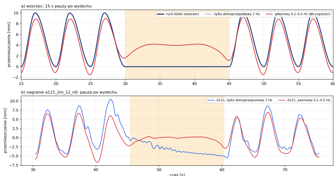
Rysunek 13.1: Pauza po wydechu po filtrze pasmowym 0,1 Hz do 0,5 Hz (czerwony) i po samym filtrze dolnoprzepustowym 2 Hz (niebieski). a) Wzorzec: filtr pasmowy przesunął pauzę w stronę połowy głębokości oddechu i dodaje pozorny ruch na jej brzegach. b) Nagranie A121 z 2 m: rzeczywista pauza z powolnym opadaniem klatki i pulsowaniem serca, które filtr pasmowy usuwa.
