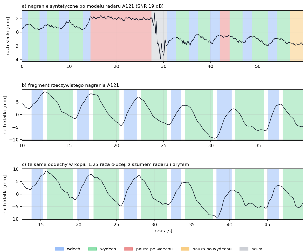
Rysunek 13.8: Dane sztuczne. a) Fragment nagrania syntetycznego: pauzy po wdechu i po wydechu oraz ruch ciała oznaczony jako szum. b) Fragment rzeczywistego nagrania A121 i c) te same oddechy w jego kopii, 1,25 raza dłuższej, z dodanym szumem radaru i dryfem. Białe przerwy to otoczenia granic wyłączone z uczenia.
