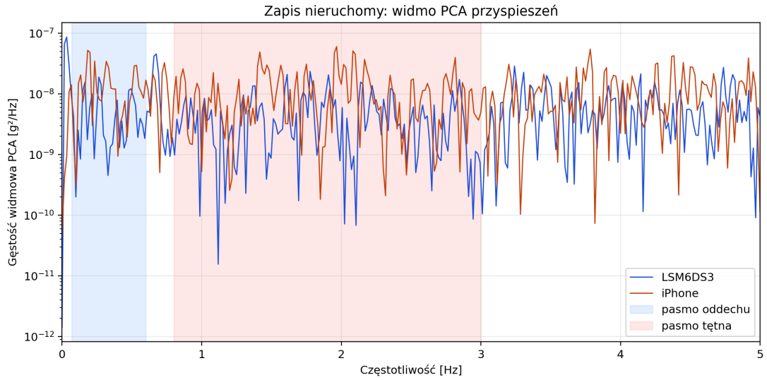
Rysunek 9.5: Gęstość widmowa pierwszej składowej PCA przyspieszeń podczas 60 s bezruchu. Zaznaczono pasmo oddechowe oraz pasmo 0,8 Hz do 3,0 Hz; nie jest to wynik detekcji tętna.
