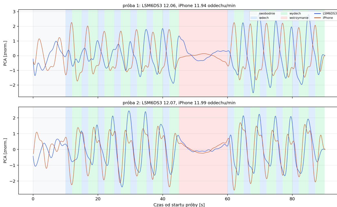
Rysunek 9.4: Znormalizowane przebiegi PCA przyspieszeń z LSM6DS3 (niebieski) i iPhone (pomarańczowy) po tej samej filtracji pasmowej 0,07 Hz do 0,60 Hz. Tło oznacza kolejne komendy programu prowadzącego. Oś czasu odnosi się do wspólnego czasu hosta; znaku i bezwzględnej amplitudy PCA nie interpretuje się fizycznie.
