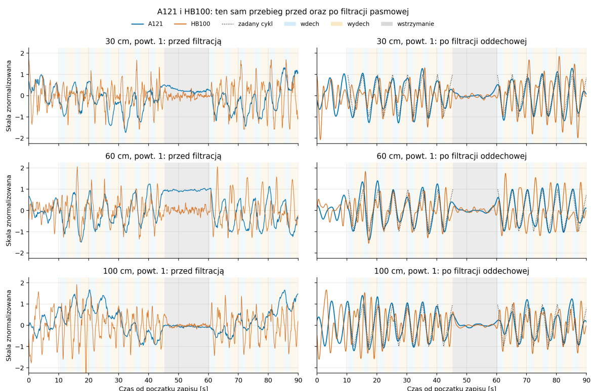
Rysunek 11.2: Przykładowe pierwsze powtórzenie na 30 cm, 60 cm i 100 cm. Lewa kolumna zawiera przebiegi przed filtracją oddechową: rozplecioną fazę IQ A121 oraz napięcie ADC HB100. Prawa pokazuje te same zapisy po filtracji pasmowej; dla A121 jest to przemieszczenie z fazy IQ, a dla HB100 napięcie IF. Sygnały znormalizowano osobno, zatem rysunek porównuje czas i kształt, nie amplitudę. Niebieskie, pomarańczowe i szare pola odpowiadają po korekcie opóźnienia odpowiednio wdechowi, wydechowi i wstrzymaniu. Drugie powtórzenia uwzględniają tabele i rysunek rytmu 11.3.
