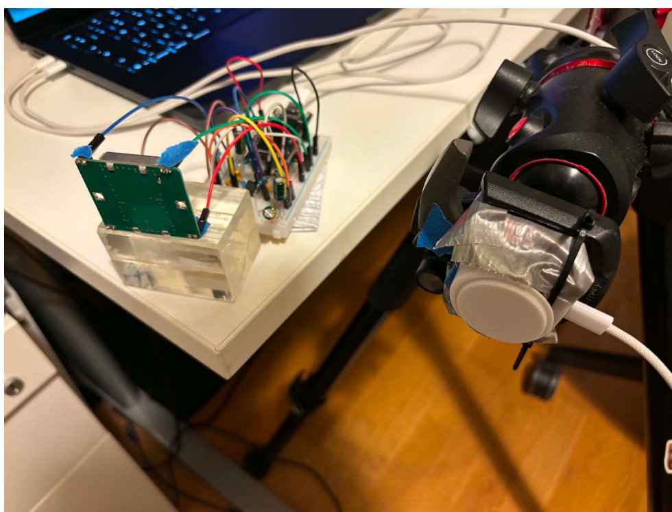
Rysunek 11.1: Elementy stanowiska równoczesnego porównania radarów: po lewej moduł HB100 z analogowym front-endem na płycie stykowej, a po prawej A121 z płaską pokrywą, zamocowany na głowicy statywu Manfrotto. Przed pomiarem położenie obu czujników korygowano do geometrii opisaną w tekście (fotografia własna).
