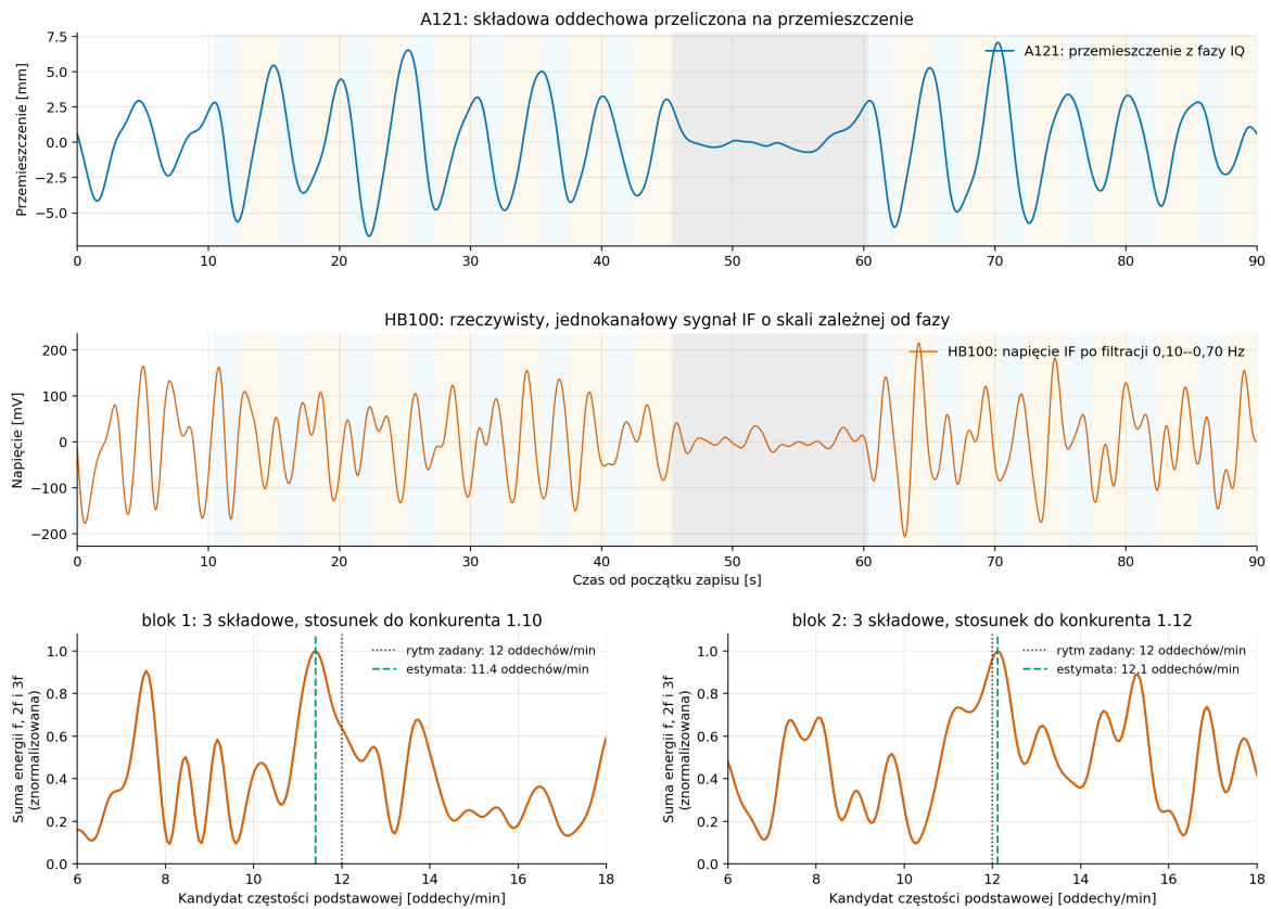
Retest 150 cm: przemieszczenie z A121 i graniczna estymacja rytmu z HB100
