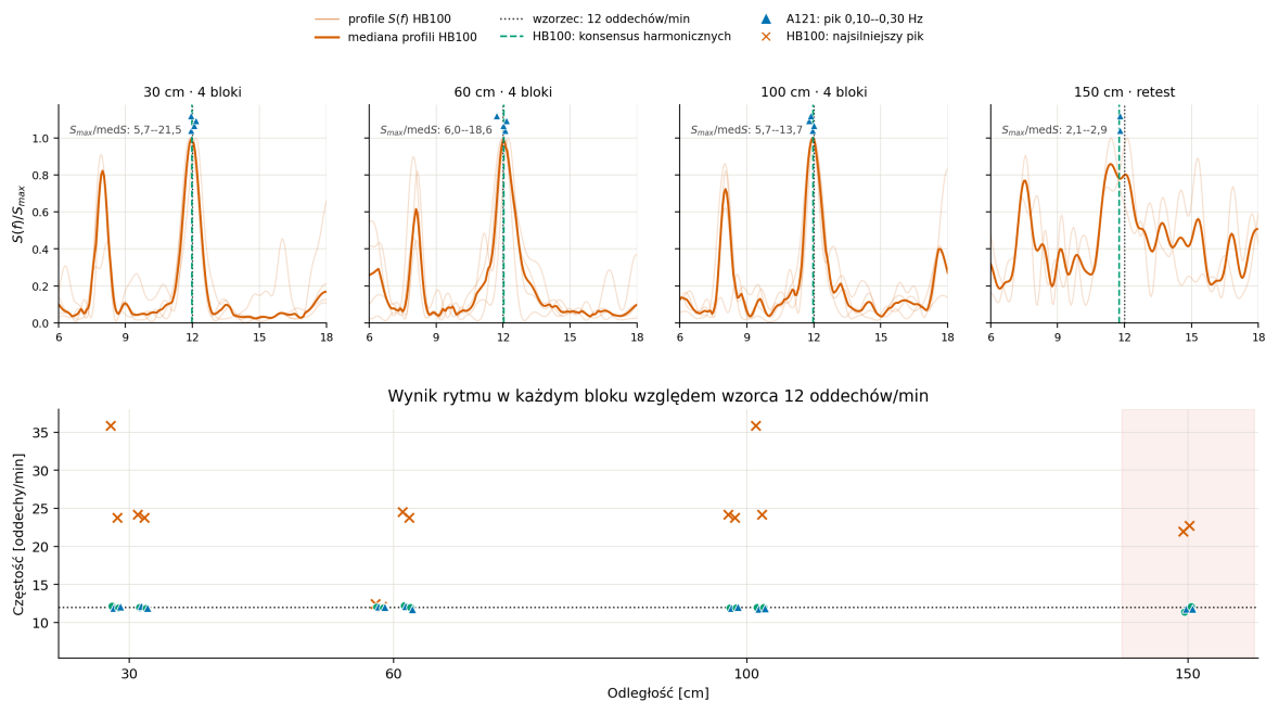
Rysunek 11.4: Porównanie estymacji rytmu we wszystkich 14 blokach. Górny rząd przedstawia funkcję konsensusu harmonicznego S(f) dla HB100: jasne linie są profilami pojedynczych bloków, ciemna — ich medianą dla danego dystansu. Linia kropkowana wyznacza zadane 12 oddechów/min, zielona — medianę estymat HB100, a niebieskie trójkąty — pik 0,10 Hz do 0,30 Hz z A121. Dolny panel pokazuje wynik każdego bloku; krzyżyki to mylące najsilniejsze piki HB100 przed złożeniem harmonicznym. Przy 30 cm do 100 cm profile HB100 mają wyraźniejszą przewagę kandydata przy 12 oddechach/min ( S_{max}/med S = 5,7-21,5 ) niż w pojedynczym reteście 150 cm (2,1-2,9).
