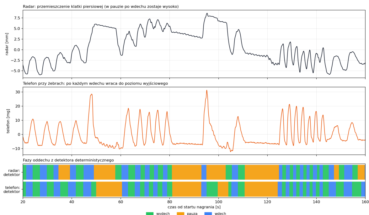
Rysunek 13.6: Fragment nagrania 3-minutowego (radar na klatkę, telefon przy żebrach). W paузach po wdechu klatka zostaje wysoko, a sygnał telefonu wraca do poziomu wyjściowego, takiego samego jak w pauzie po wydechu (111 s–125 s); dlatego pauzy po wdechu i po wydechu połączono w jedną klasę.
