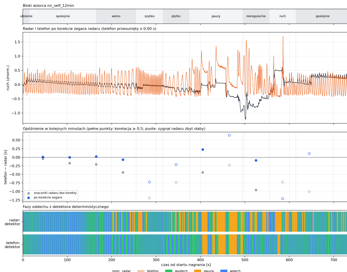
Rysunek 13.5: Nagranie nn_self_12min leżąc, radar pod kątem, telefon po drugiej stronie. Od góry: bloki wzorca, sygnały po korekcie zegara radaru, opóźnienie telefon – radar w kolejnych minutach przed korektą i po niej (puste punkty: za słaby sygnał radaru) oraz fazy z detektora na radarze i na telefonie.
