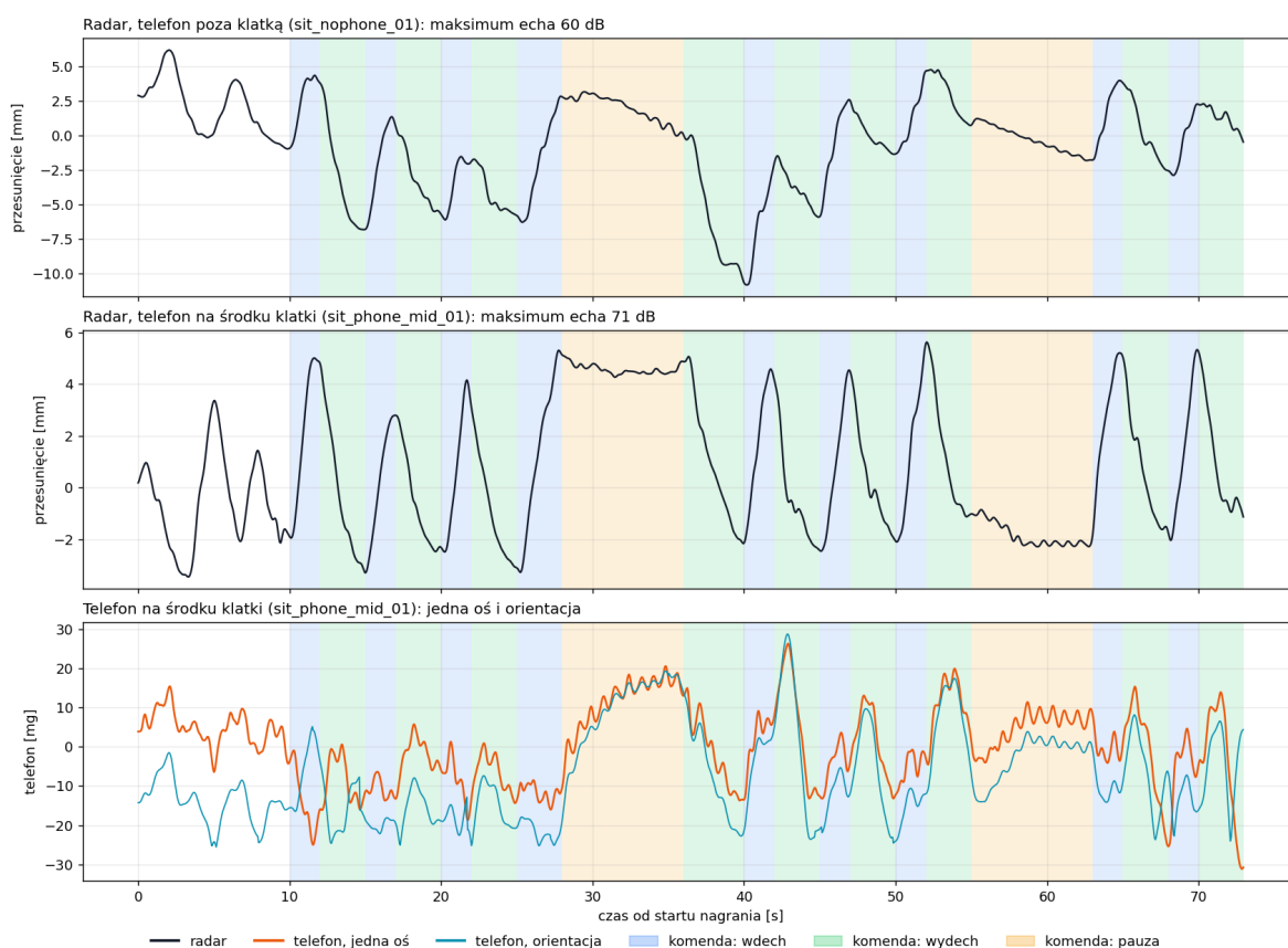
Rysunek 13.9: Ta sama pozycja, dwie kolejne próby z komendami (tło). U góry radar bez telefonu na klatce, w środku radar z telefonem na środku klatki ekranem do radaru (echo o 10 dB silniejsze, przebieg gładzszy, bo radar widzi głównie telefon), u dołu przebieg samego telefonu na mostku: zaszumiony i dryfujący w pauzach.
