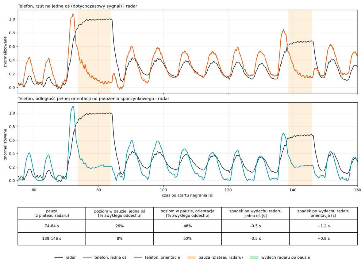
Rysunek 13.8: Nagranie, na którym sygnału orientacji nie opracowywano ( phase1_halfside_02 ); pauzy (tło) wyznaczył detektor na radarze. Sygnał jednoosiowy (u góry) opada do poziomu wyjściowego przed końcem obu pauz po głębokim wdechu; orientacja (u dołu) zostaje na mniej więcej połowie zwykłego oddechu i spada razem z wydechem radaru.
