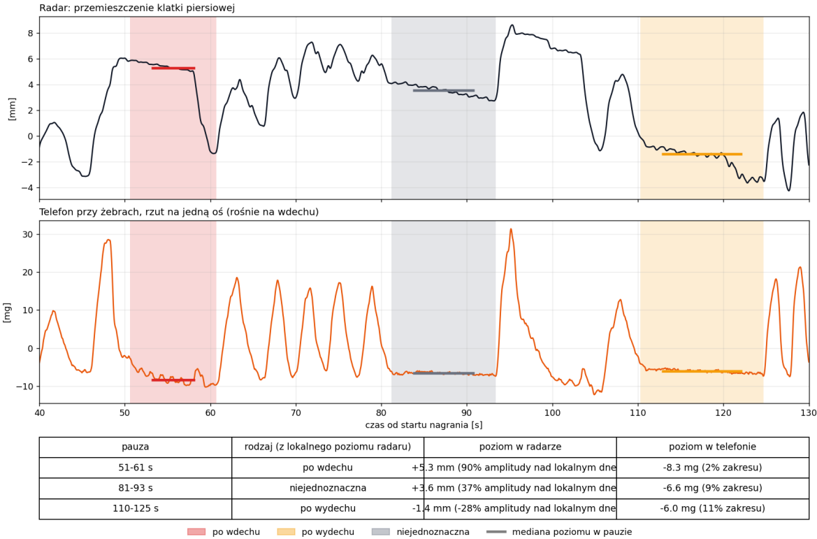
Rysunek 13.6: Trzy pauzy w nagraniu 3-minutowym (radar na klatkę, telefon przy żebrach); poziom w pauzie to mediana bez 2,5s przy krawędziach, rodzaj pauzy z lokalnego poziomu radaru. Radar pokazuje poziom klatki, a telefon (rzut na jedną oś) w każdej z pauz wraca do tego samego poziomu wyjściowego, dlatego pauzy po wdechu i po wydechu połączono w jedną klasę.
