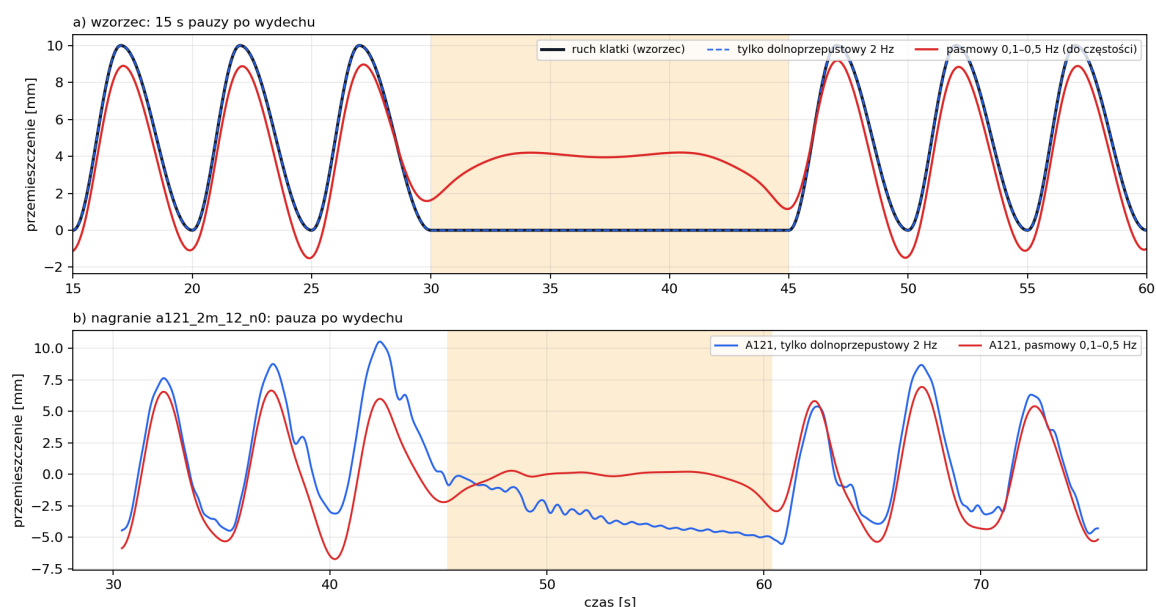
Rysunek 13.1: Pauza po wydechu po filtrze pasmowym 0,1 Hz do 0,5 Hz (czerwony) i po samym filtrze dolnoprzepustowym 2 Hz (niebieski). a) Wzorzec: filtr pasmowy przesuwą pauzę w stronę połowy głębokości oddechu i dodaje pozorny ruch na jej brzegach. b) Nagranie A121 z 2 m: rzeczywista pauza z powolnym opadaniem klatki i pulsowaniem serca, które filtr pasmowy usuwa.
