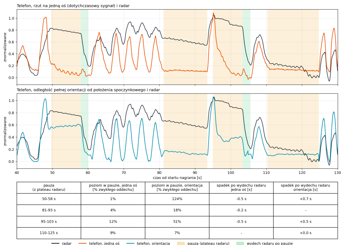
Rysunek 13.7: Te same pauzy w nagraniu 3-minutowym: u góry dotychczasowy sygnał z telefonu (rzut przyspieszenia na jedną oś), u dołu odległość pełnej orientacji telefonu (nachylenia w dwóch kierunkach) od położenia spoczynkowego, które wyznaczają dna poprzednich oddechów. Czarna linia to radar, zielone tło to wydech radaru po pauzie. W pauzach po głębokim wdechu (50 s do 58 s, 95 s do 103 s) orientacja utrzymuje poziom i spada razem z wydechem radaru (po +0,7 i +0,5 s), a sygnał jednoosiowy wraca do poziomu wyjściowego jeszcze przed końcem pauzy (ujemny czas w tabeli); w pauzie po wydechu (110 s do 125 s) obie wielkości zostają przy dole. Wynik wstępny: jedno nagranie, to samo, na którym efekt zauważono, bez niezależnej weryfikacji.
