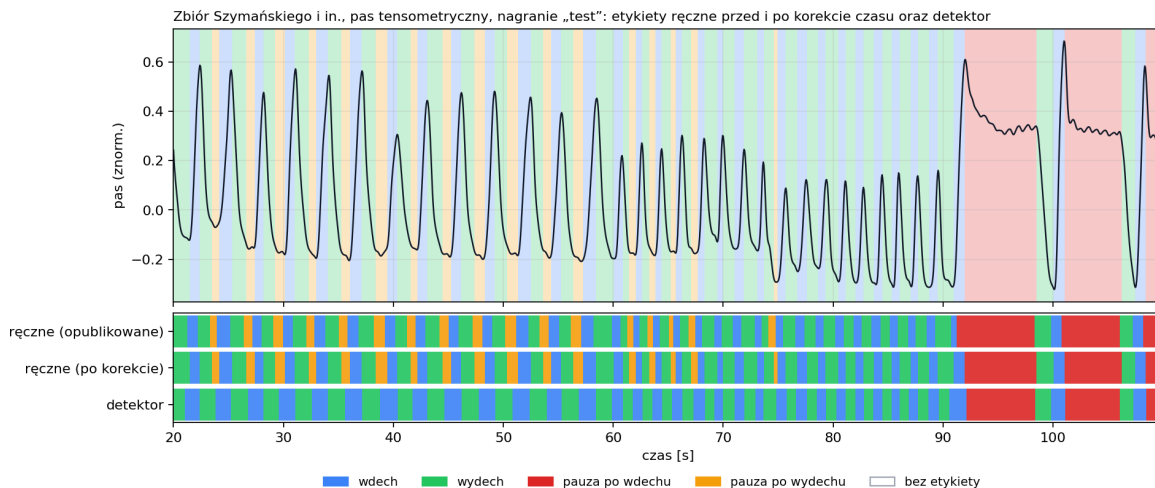
Rysunek 13.11: Nagranie pasa ze zbioru [26]. Tło: etykiety ręczne po korekcie czasu; paski: etykiety opublikowane, po korekcie i detektor deterministyczny. Po korekcie granice leżą na zwrotach pasa, a pauza po wdechu zaczyna się w szczycie; szybkie osiadanie tuż po nim należy do pauzy, zarówno w etykietach, jak i w detektorze. Krótkie pauzy po wydechu detektor wlicza do wydechu.
