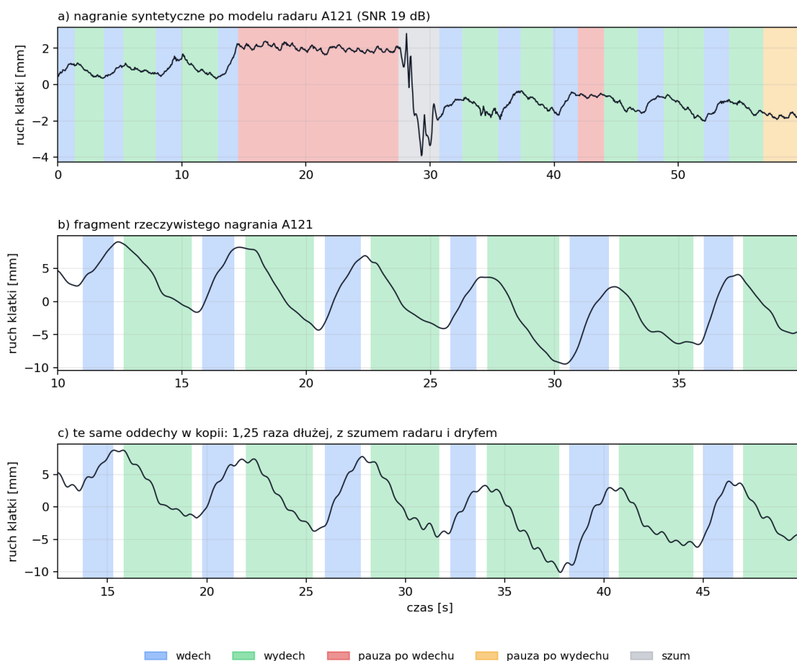
Rysunek 13.12: Dane sztuczne. a) Fragment nagrania syntetycznego: pauzy po wdechu i po wydechu oraz ruch ciała oznaczony jako szum. b) Fragment rzeczywistego nagrania A121 i c) te same oddechy w jego kopii, 1,25 raza dłuższej, z dodanym szumem radaru i dryfem. Białe przerwy to otoczenia granic wyłączone z uczenia.
