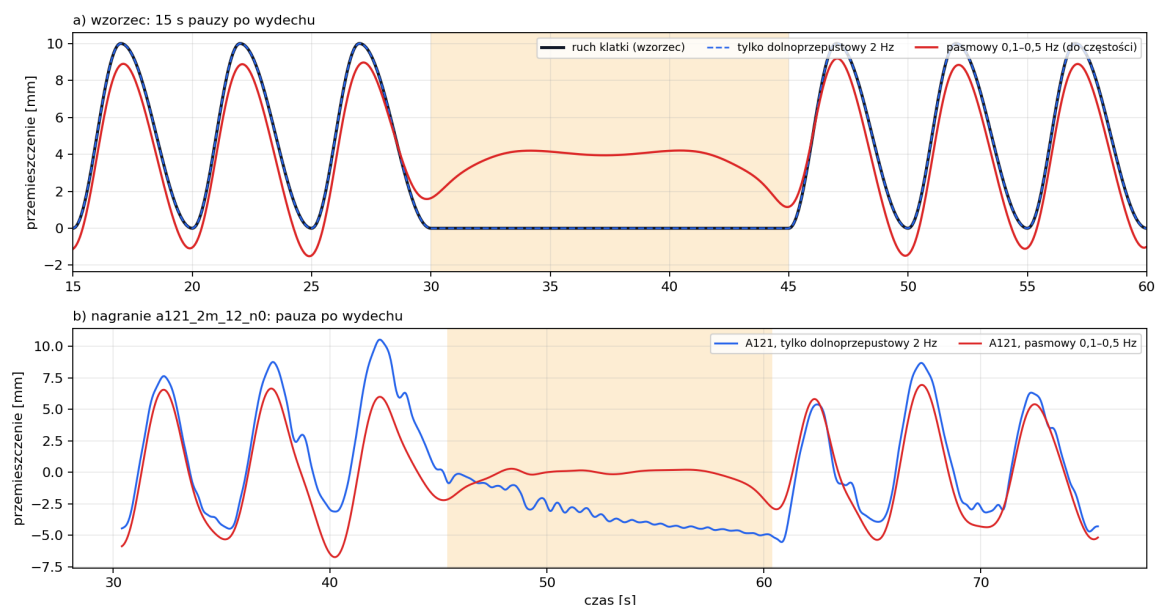
Rysunek 13.1: Pauza po wydechu po filtrze pasmowym 0,1 Hz do 0,5 Hz (czerwony) i po samym filtrze dolnoprzepustowym 2 Hz (niebieski). a) Wzorzec: filtr pasmowy przesuwają pauzę w stronę połowy głębokości oddechu i dodaje pozorny ruch na jej brzegach. b) Nagranie A121 z 2 m: rzeczywista pauza z powolnym opadaniem klatki i pulsowaniem serca, które filtr pasmowy usuwa.
