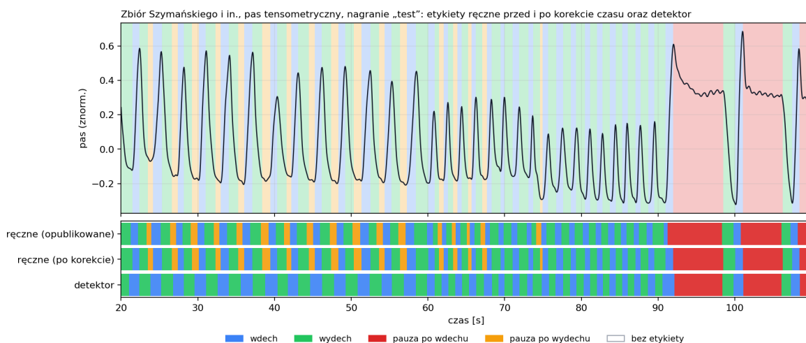
Rysunek 13.6: Nagranie pasa ze zbioru [26]. Tło: etykiety ręczne po korekcie czasu; paski: etykiety opublikowane, po korekcie i detektor deterministyczny. Po korekcie granice leżą na zwrotach pasa, a pauza po wdechu zaczyna się w szczycie; szybkie osiadanie tuż po nim należy do pauzy, zarówno w etykietach, jak i w detektorze. Krótkie pauzy po wydechu detektor wlicza do wydechu.
