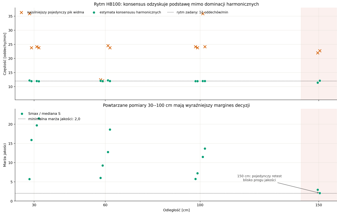
Rysunek 11.5: Estymacja rytmu HB100 we wszystkich 14 blokach. Krzyżyki oznaczają najsilniejszy pojedynczy pik widma, a zielone punkty — wynik konsensusu harmonicznych; każdy pomiar zawiera dwa bloki. W powtarzanej serii 30 cm do 100 cm wszystkie 12 estymat mieszczą się w zakresie 11,9–12,2 oddechów/min wobec zadanych 12 oddechów/min. Dwa punkty przy 150 cm należą do pojedynczego retestu i leżą blisko progu jakości S_{\max}/\text{med } S = 2,0 ; nie stanowią potwierdzenia użytecznej estymacji faz oddechu.
