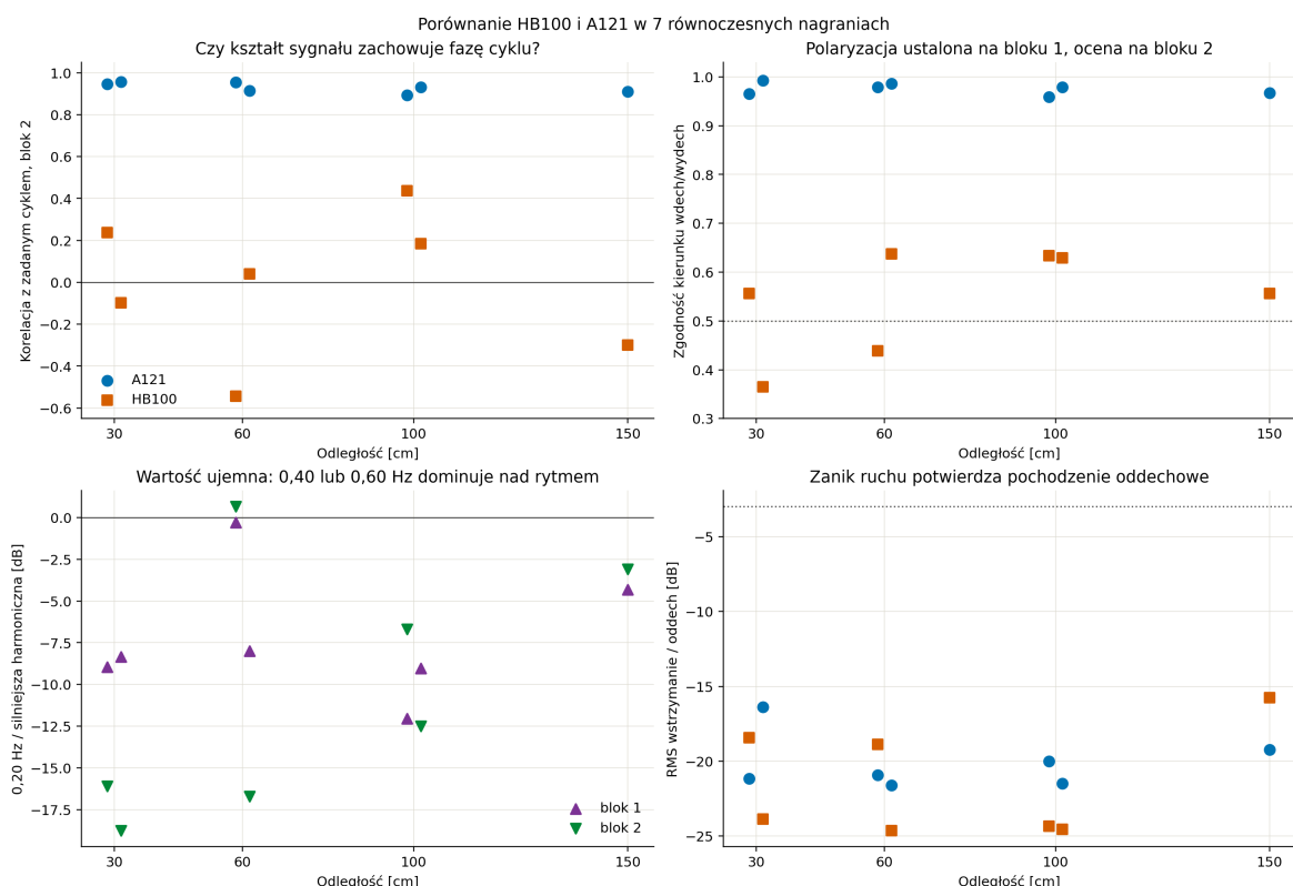
Rysunek 11.6: Metryki sześciu prób podstawowych oraz pojedynczego retestu 150 cm. Dwa górne panele dotyczą drugiego bloku po kalibracji polaryzacji na pierwszym. Lewy dolny panel pokazuje poziom składowej 0,20 Hz względem silniejszej z harmonicznych 0,40 Hz i 0,60 Hz; wartość ujemna oznacza dominację harmoniczną. Prawy dolny panel przedstawia zanik RMS podczas wstrzymania; linia kropkowana wskazuje próg -3 dB. Przesunięcie punktów wokół dystansu rozróżnia dwa powtórzenia.
