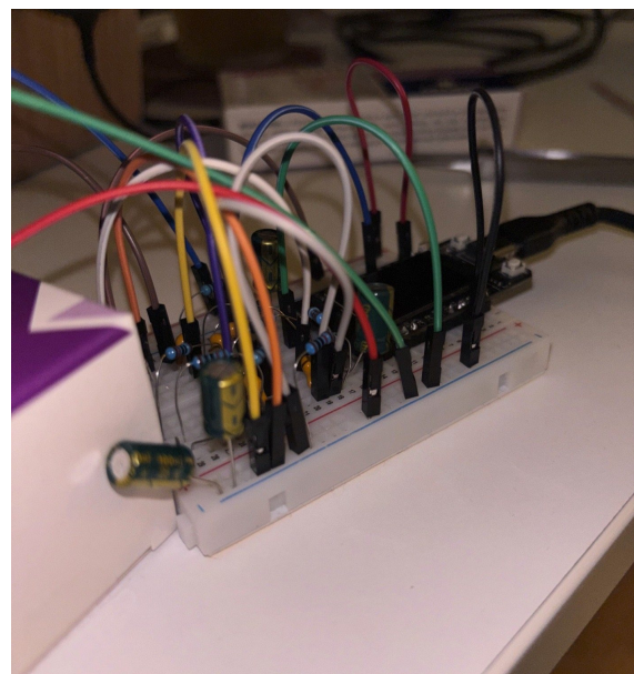
(b) Zbliżenie analogowego front-endu na płytce stykowej.
