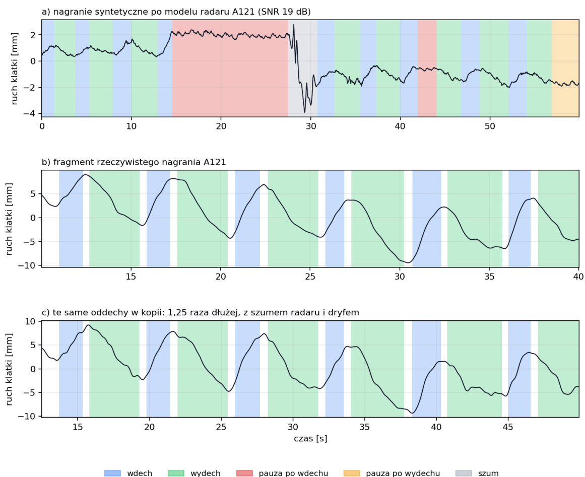
Rysunek 13.6: Dane sztuczne. a) Fragment nagrania syntetycznego: pauzy po wdechu i po wydechu oraz ruch ciała oznaczony jako szum. b) Fragment rzeczywistego nagrania A121 i c) te same oddechy w jego kopii, 1,25 raza dłuższej, z dodanym szumem radaru i dryfem. Białe przerwy to otoczenia granic wyłączone z uczenia.
