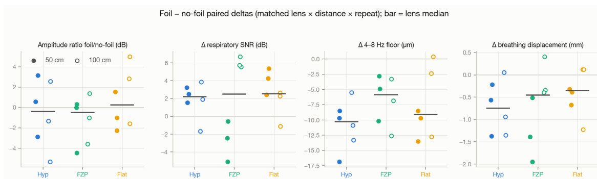
Rysunek 11.5: Parowane różnice folia – brak folii po dopasowaniu soczewki, dystansu i numeru powtórzenia. Każdy punkt jest jedną parą; punkty wypełnione oznaczają 50 cm, puste 100 cm, pozioma kreska — medianę dla soczewki, a linia zera — brak zmiany. Dodatnia wartość oznacza wzrost danej metryki z folią; w panelu szumu wartość ujemna jest więc korzystna. Amplituda oscyluje wokół zera, natomiast podobny dla wszystkich soczewek spadek szumu jest sygnaturą różnicy sesji, a nie selektywnego działania reflektora.
