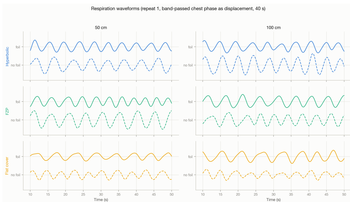
Rysunek 11.6: 40 sekund przefiltrowanego sygnału przemieszczenia klatki piersiowej (fragment 10s do 50s) z pierwszego powtórzenia każdego z 12 warunków. Wiersze odpowiadają soczewkom, kolumny dystansom, linia ciągła oznacza folię, a przerywana jej brak. Przebiegi przesunięto pionowo, aby się nie nakładały, dlatego ich poziom zerowy nie ma znaczenia; porównywać należy amplitudę i regularność. Wszystkie są czytelne, lecz płaska pokrywa daje wyraźnie mniejszą amplitudę ruchu.
