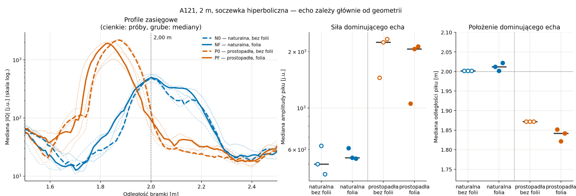
Rysunek 11.8: Profile zasięgowe i echo przy 2 m. W lewym panelu cienka krzywa jest medianą po czasie z jednej próby, a gruba medianą trzech prób; linie niebieskie oznaczają pozycję naturalną, pomarańczowe prawie prostopadłą, ciągłe folię, a przerywane jej brak. Linia pionowa wskazuje dystans nominalny ustawiony dalmierzem. Środkowy panel pokazuje medianową amplitudę dominującego piku, prawy jego położenie; punkty to próby, a czarne kreski mediany warunków.
