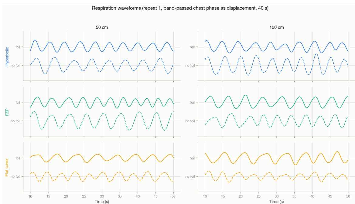
Rysunek 11.6: 40 sekund przefiltrowanego sygnału przemieszczenia klatki piersiowej dla każdego z 12 warunków. Wszystkie przebiegi są czytelne; przebiegi z płaską pokrywą mają wyraźnie mniejszą amplitudę.
