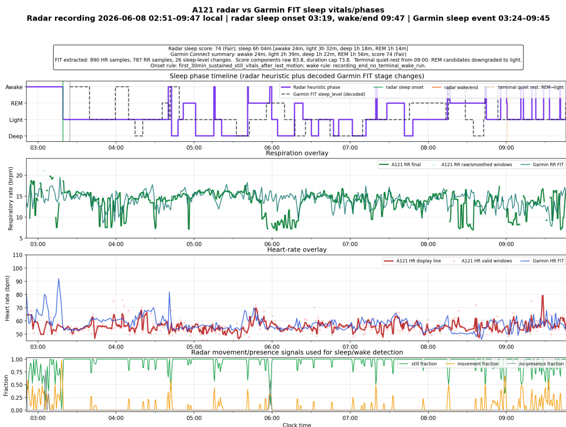
Rysunek 13.1: Noc 1 (soczewka plano-convex). Tętno i oddech z radaru oraz heurystyczne fazy snu nałożone na dane referencyjne z Garmina.
