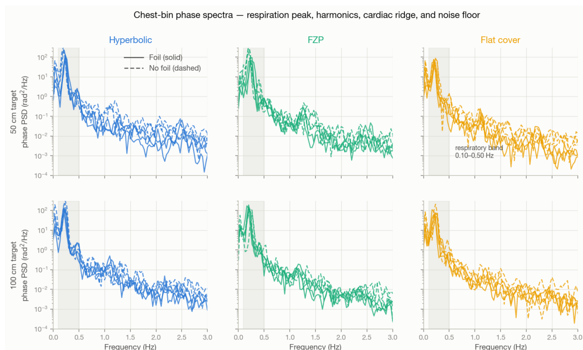
Rysunek 11.3: Widma gęstości mocy sygnału fazowego z bramek klatki piersiowej. Każde nagranie wykazuje tę samą strukturę: dominujący pik oddechowy w zacie-nionym paśmie, harmoniczne oraz szumowe tło. Wybór soczewki niemal nie zmienia odległości piku od tła.
