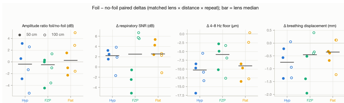
Rysunek 11.5: Parowane różnice folia – brak folii. Amplituda oscyluje wokół zera; spadek szumu ruchowego jest jednorodny dla wszystkich soczewek — sygnatura efektu sesji, a nie efektu reflektora.
