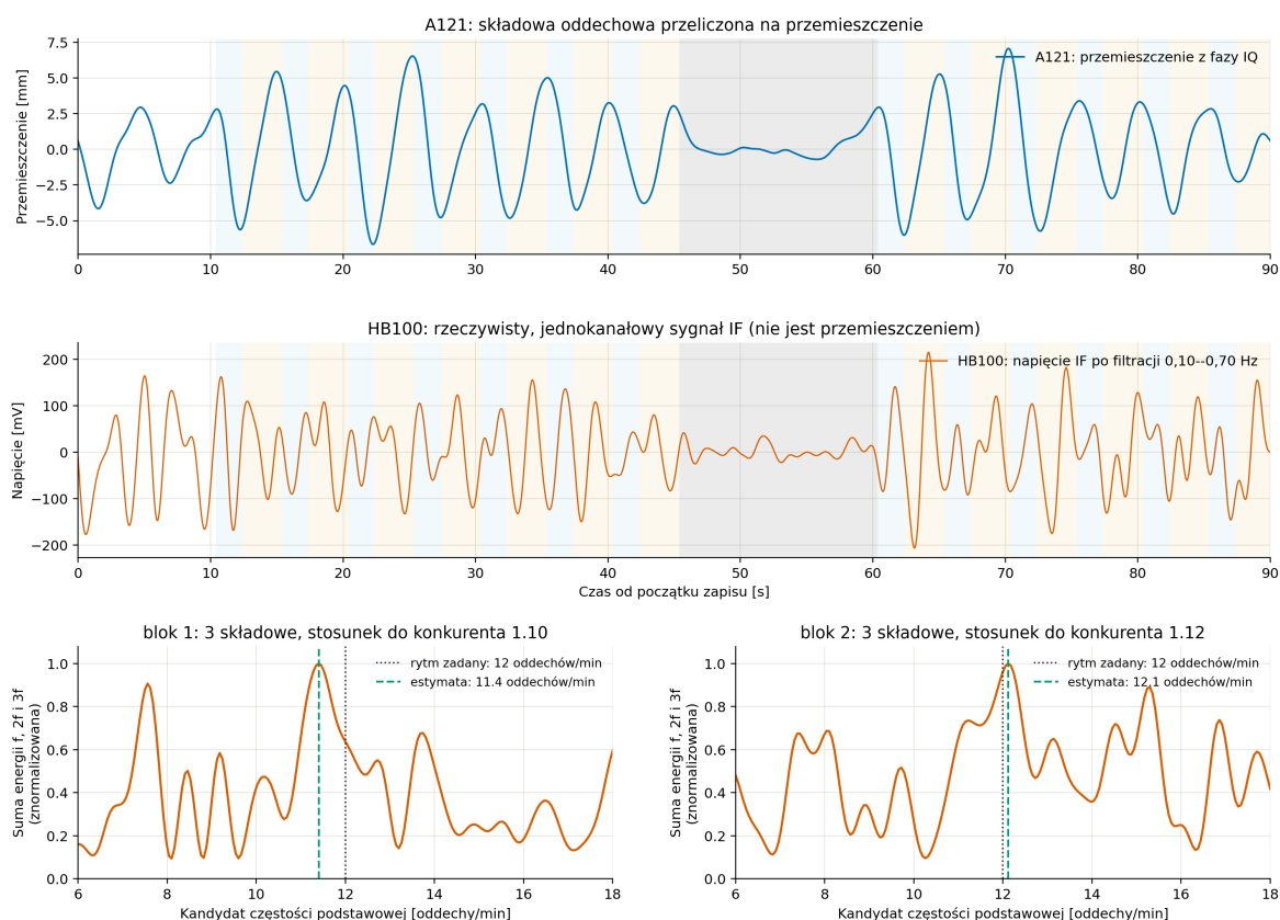
Rysunek 11.4: Pojedynczy retest na 150 cm. Górny panel pokazuje przemieszczenie wyznaczone z fazy IQ A121, środkowy — jednokanałowe napięcie IF HB100; zachowano osobne jednostki, aby nie sugerować ich równoważności. Dolne panele pokazują funkcję (11.2): mimo najsilniejszych pików napięcia przy około 0,37 Hz, estymator wskazał 0,190 Hz (11,4 oddechów/min) oraz 0,202 Hz (12,1 oddechów/min) wobec zadanego rytmu 0,20 Hz. Nie nadaje to sygnałowi HB100 kierunku wdech–wydech.
