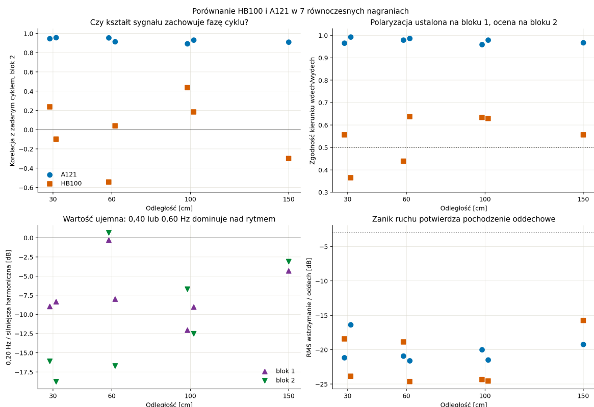
Rysunek 11.5: Metryki sześciu prób podstawowych oraz pojedynczego retestu 150 cm. Dwa górne panele dotyczą drugiego bloku po kalibracji polaryzacji na pierwszym. Lewy dolny panel pokazuje poziom składowej 0,20 Hz względem silniejszej z harmonicznych 0,40 Hz i 0,60 Hz; wartość ujemna oznacza dominację harmoniczną. Prawy dolny panel przedstawia zanik RMS podczas wstrzymania; linia kropkowana wskazuje próg -3 dB. Przesunięcie punktów wokół dystansu rozróżnia dwa powtórzenia.
