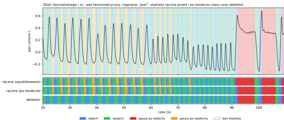
Rysunek 13.8: Nagranie pasa ze zbioru [26]. Tło: etykiety ręczne po korekcie czasu; paski: etykiety opublikowane, po korekcie i detektor deterministyczny. Po korekcie granice leżą na zwrotach pasa, a pauza po wdechu zaczyna się w szczycie; szybkie osiadanie tuż po nim należy do pauzy, zarówno w etykietach, jak i w detektorze. Krótkie pauzy po wydechu detektor wlicza do wydechu.
