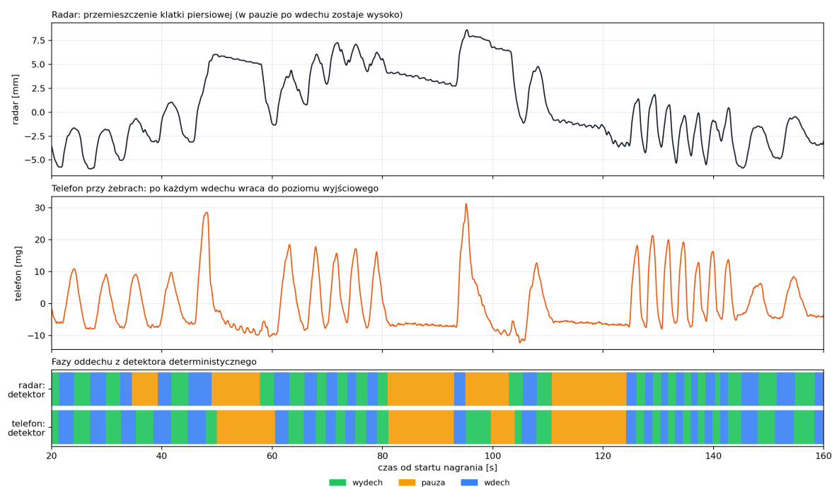
Rysunek 13.6: Fragment nagrania 3-minutowego (radar na klatkę, telefon przy żebrach). W pauzach po wdechu klatka zostaje wysoko, a sygnał telefonu wraca do poziomu wyjściowego, takiego samego jak w pauzie po wydechu (111s–125s); dlatego pauzy po wdechu i po wydechu połączono w jedną klasę.
