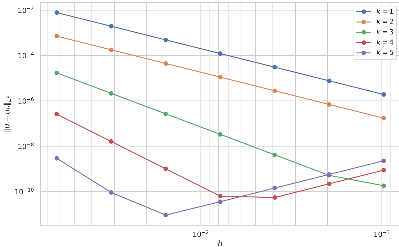
Item (g): erro de u_h com \delta_1 = -1/2 e \beta = 0
