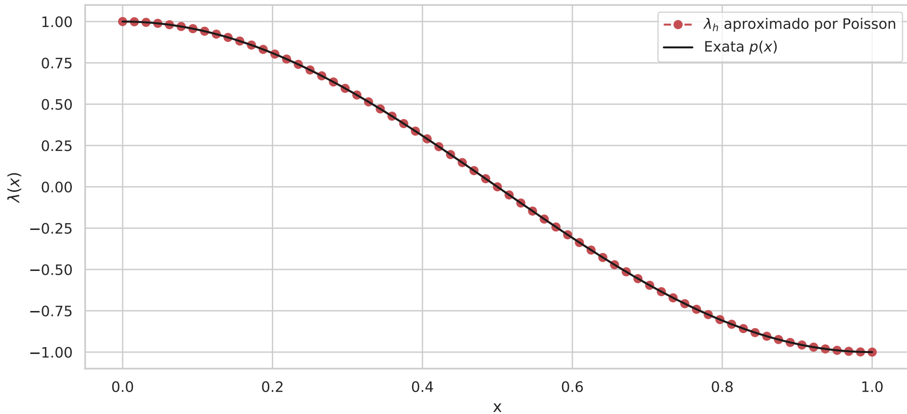
Item (i): aproximação de \lambda = p , N = 64 , k = 1
