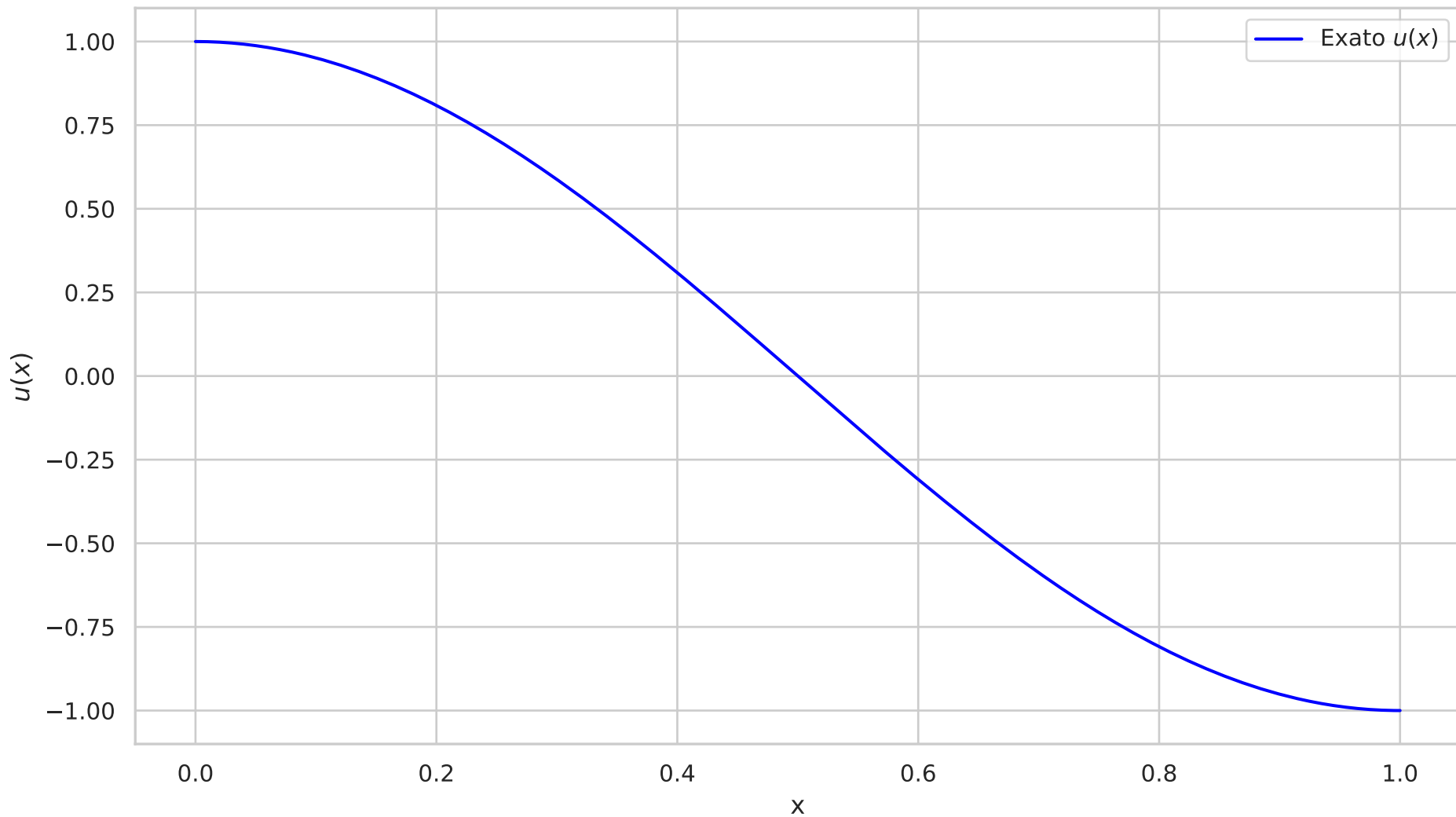
Solução exata u(x) = \cos(\pi x)
