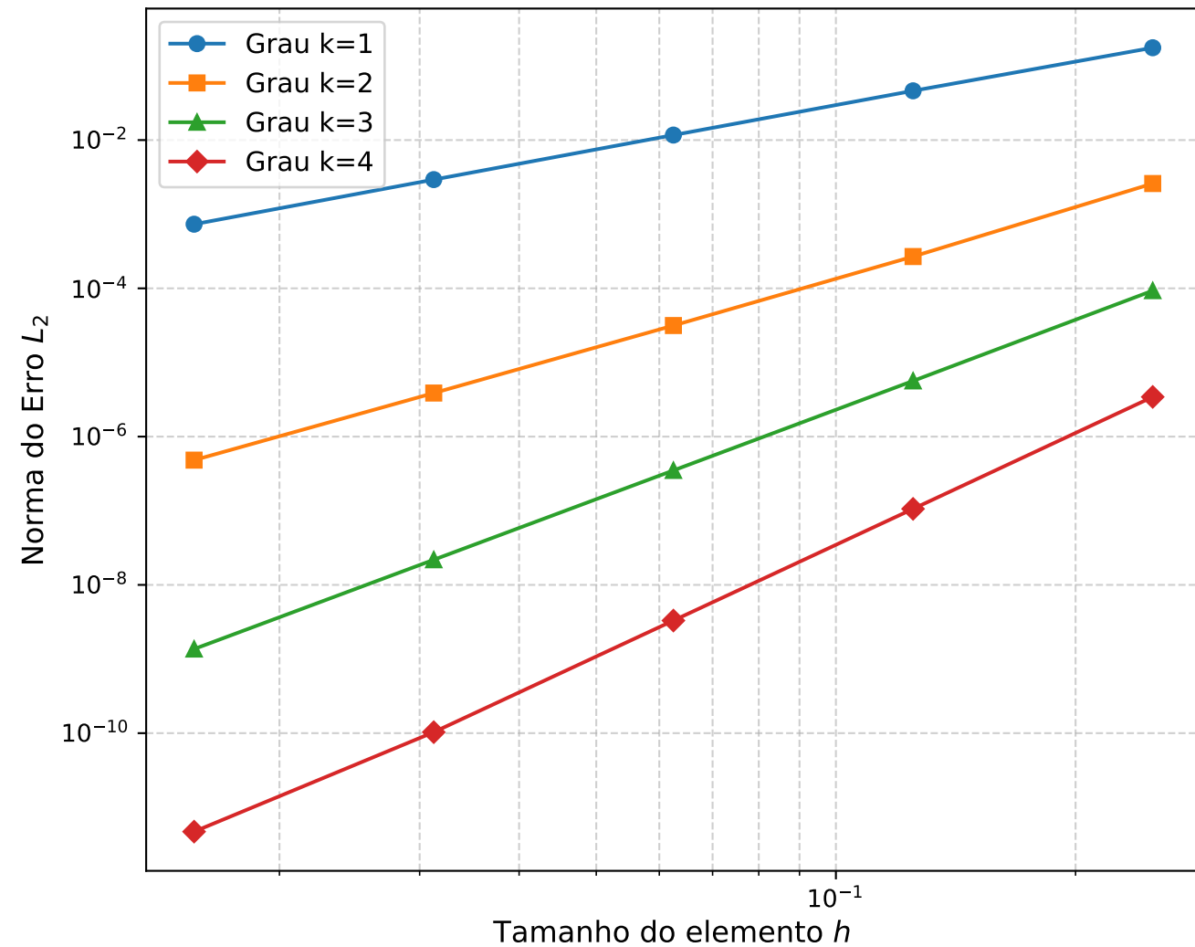
Convergência L2 - Variável p
