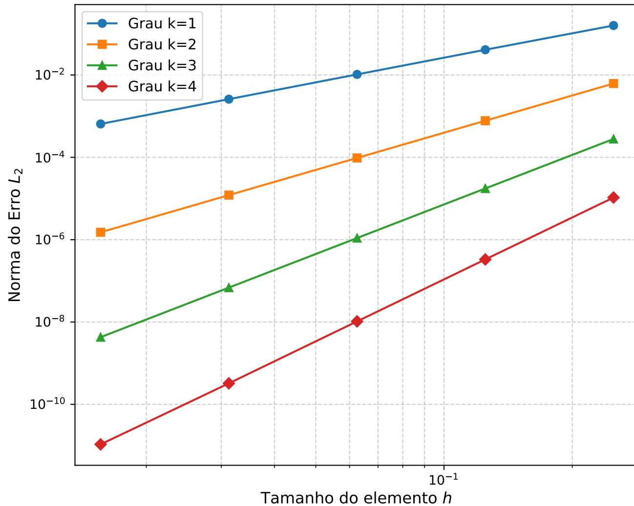
Convergência L2 - Variável u
