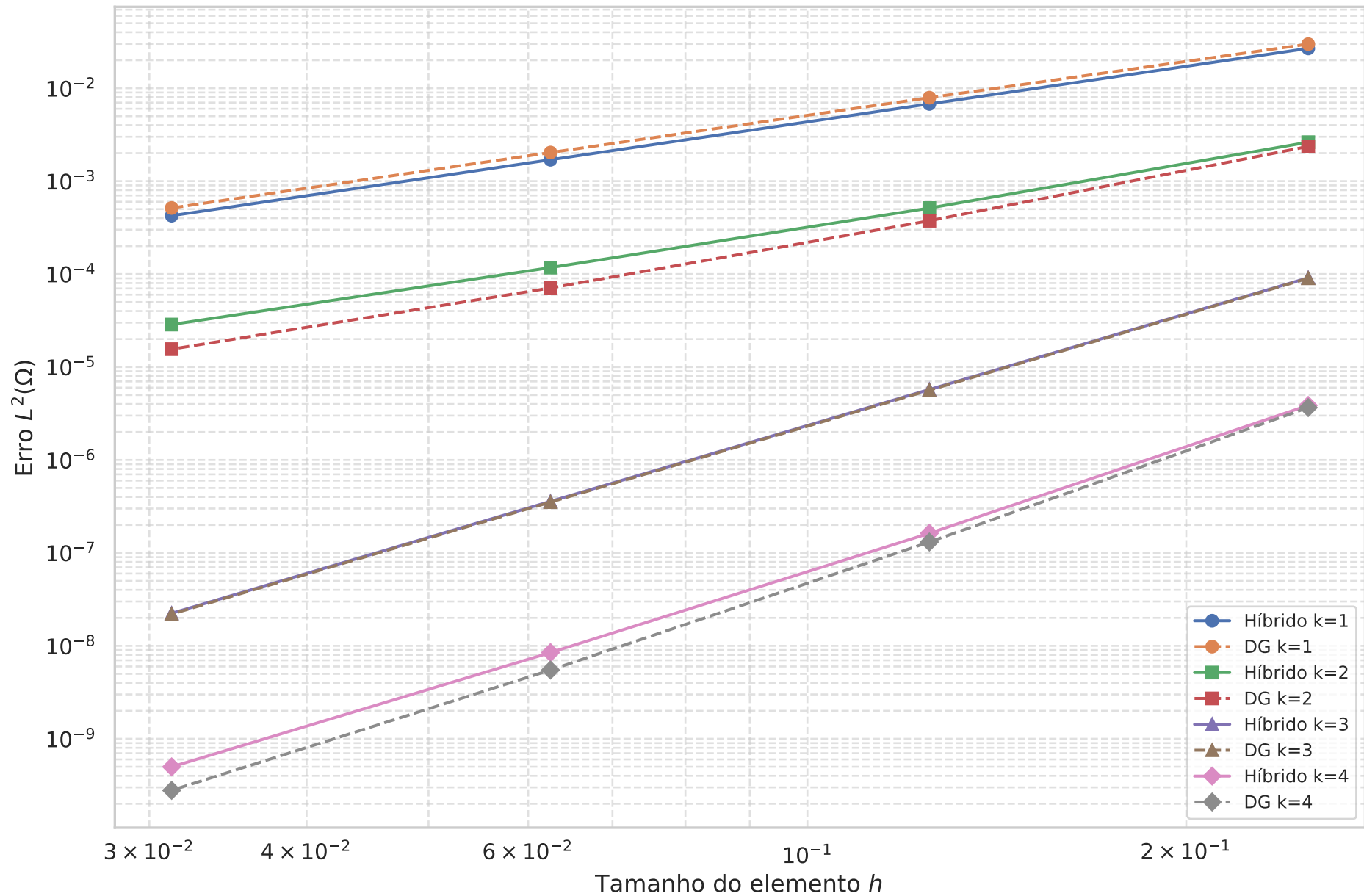
Erro L^2 - Híbrido vs DG, \alpha = 0
