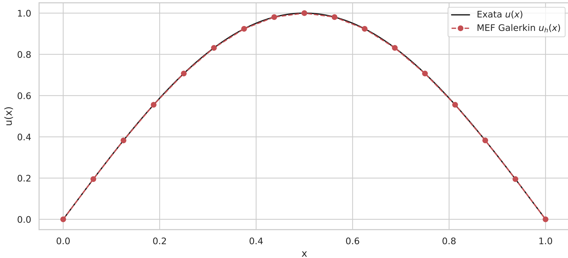
Galerkin clássico: N = 16 , k = 1
