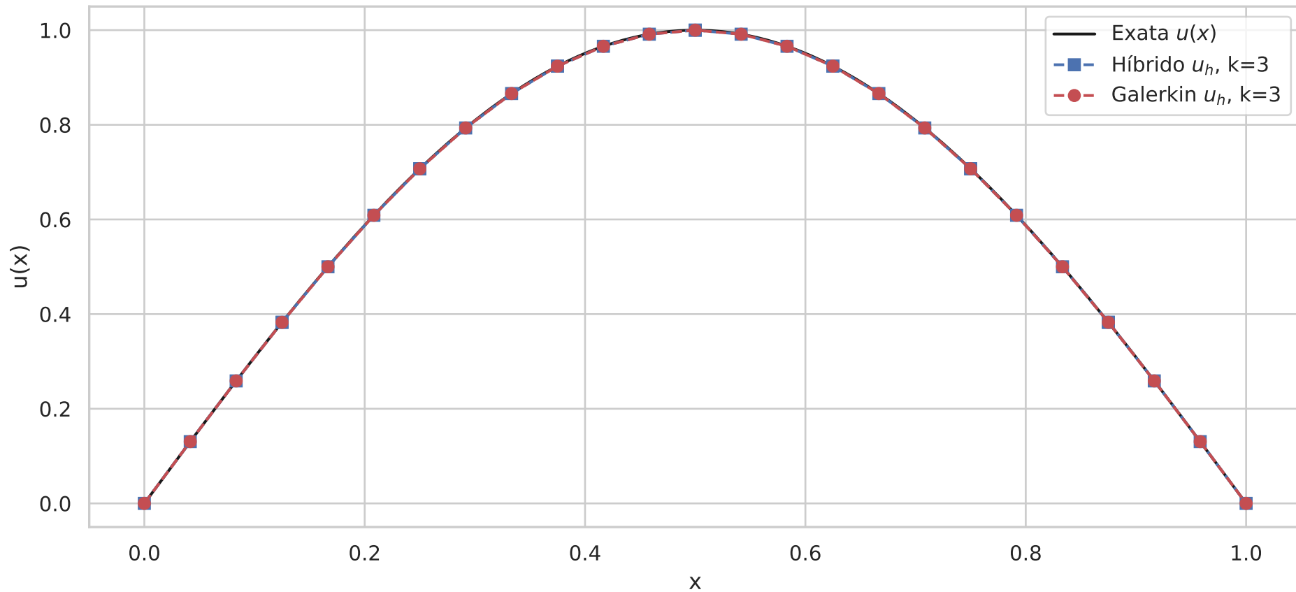
Comparação das soluções, \alpha = -1 , \beta = 7.20e + 02
